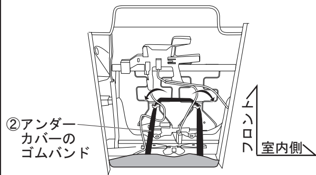
〈シートクッション裏側図〉
