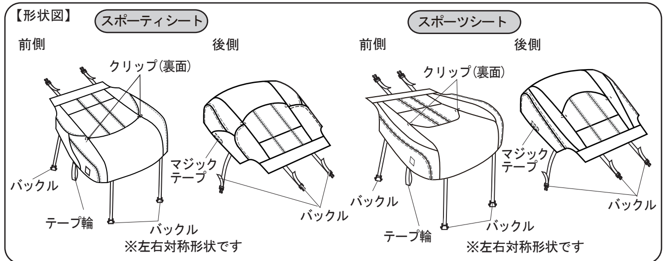
〈シートクッション裏側図〉
