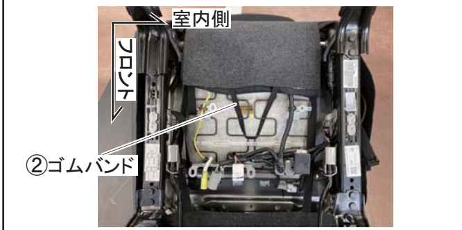
〈フロントシートクッション裏側図〉
