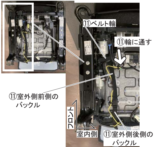
〈フロントシートクッション裏側室内側図〉
