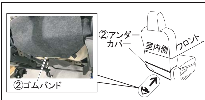
〈フロントシートクッション裏側図〉
