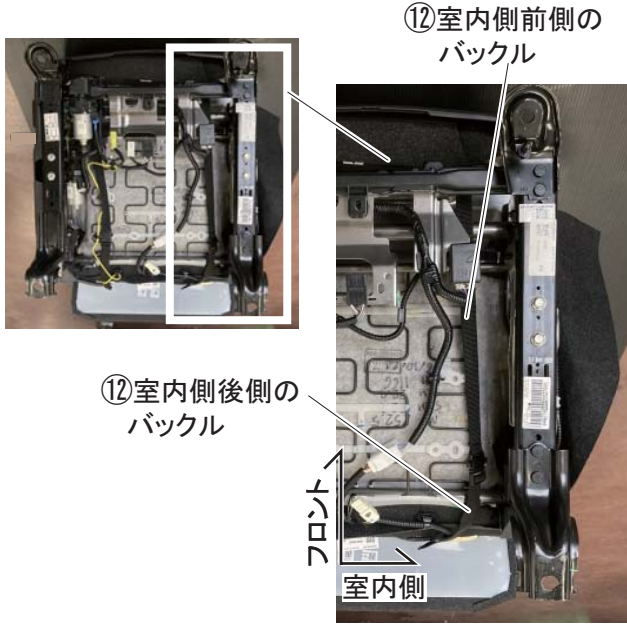
〈フロントシートクッション裏側室内側図〉
