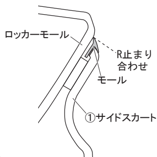
A-A 断面図
