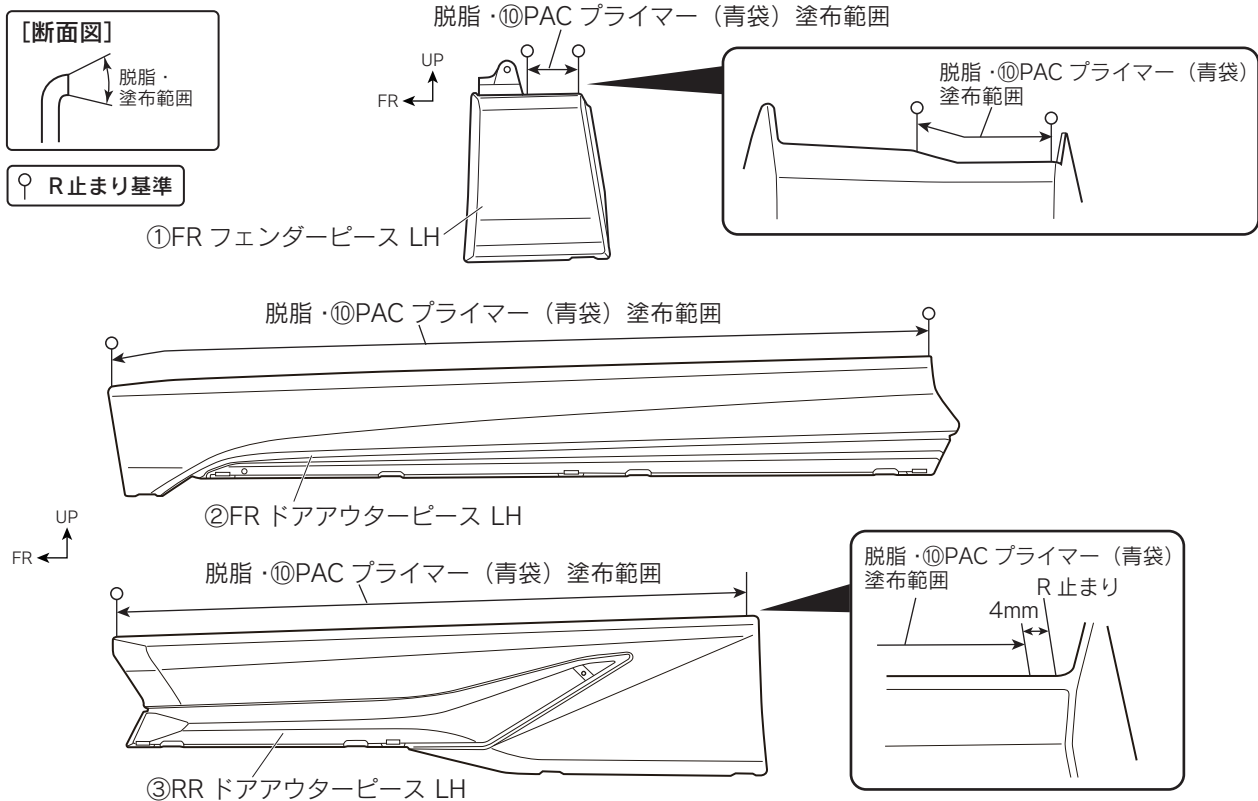
図 28 ※L H 図示 左右共通作業
