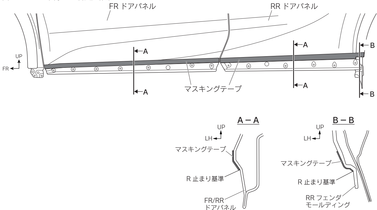
図5 ※LH図示 左右共通作業
