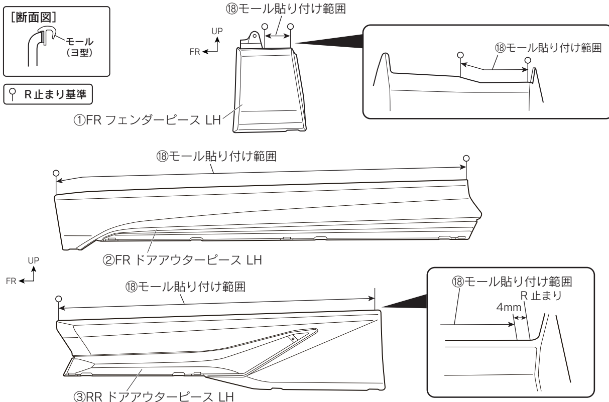
図 29 ※ L H 図示 左右共通作業
