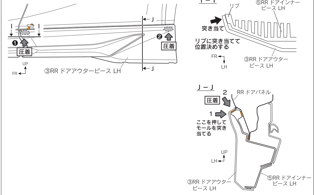
図 24 ※ L H 図示 左右共通作業
