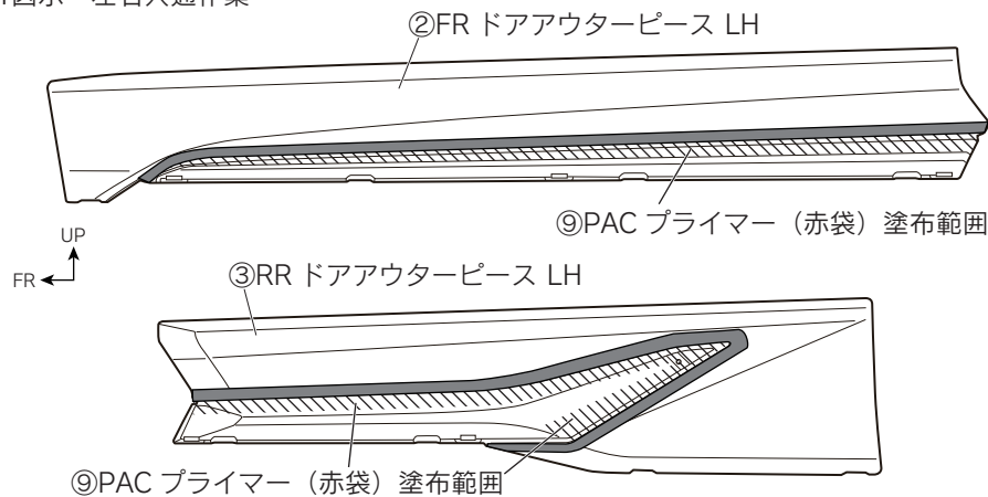
図 33 ※LH図示 左右共通作業
