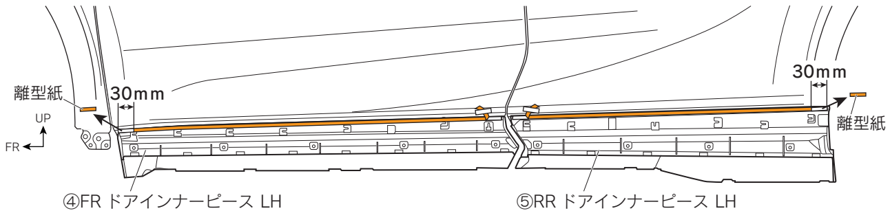
図 18 ※LH 図示 左右共通作業
