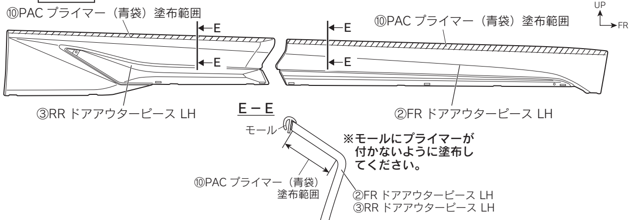
図 16 裏面視 ※LH図示 左右共通作業
