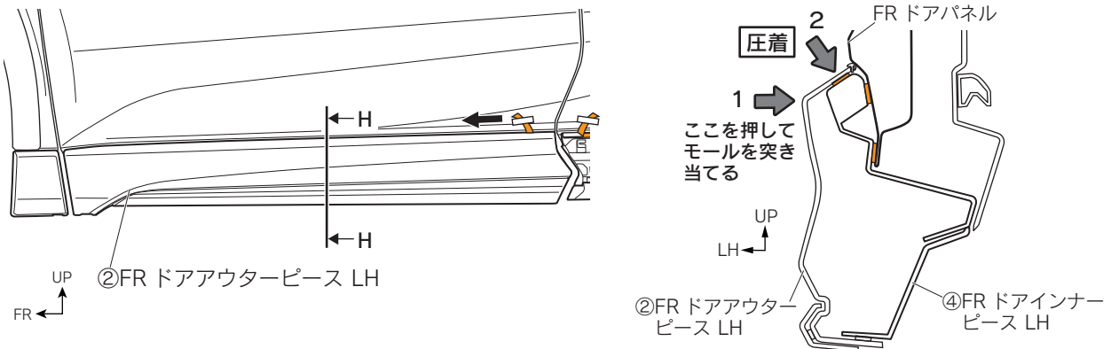
図 22 ※L H図示 左右共通作業
