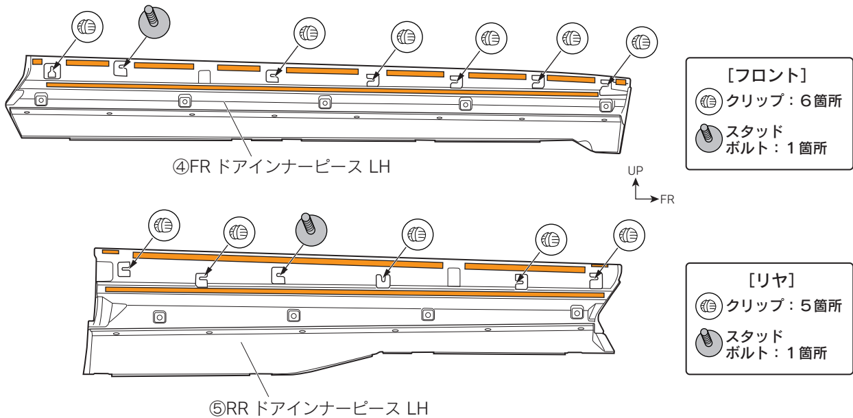
図4 裏面視 ※LH図示 左右共通作業
