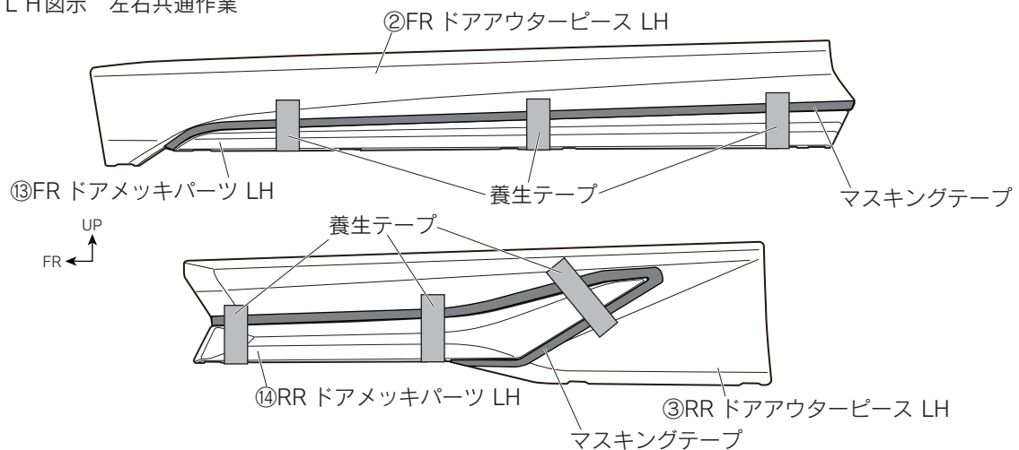
図 31 ※LH図示 左右共通作業
