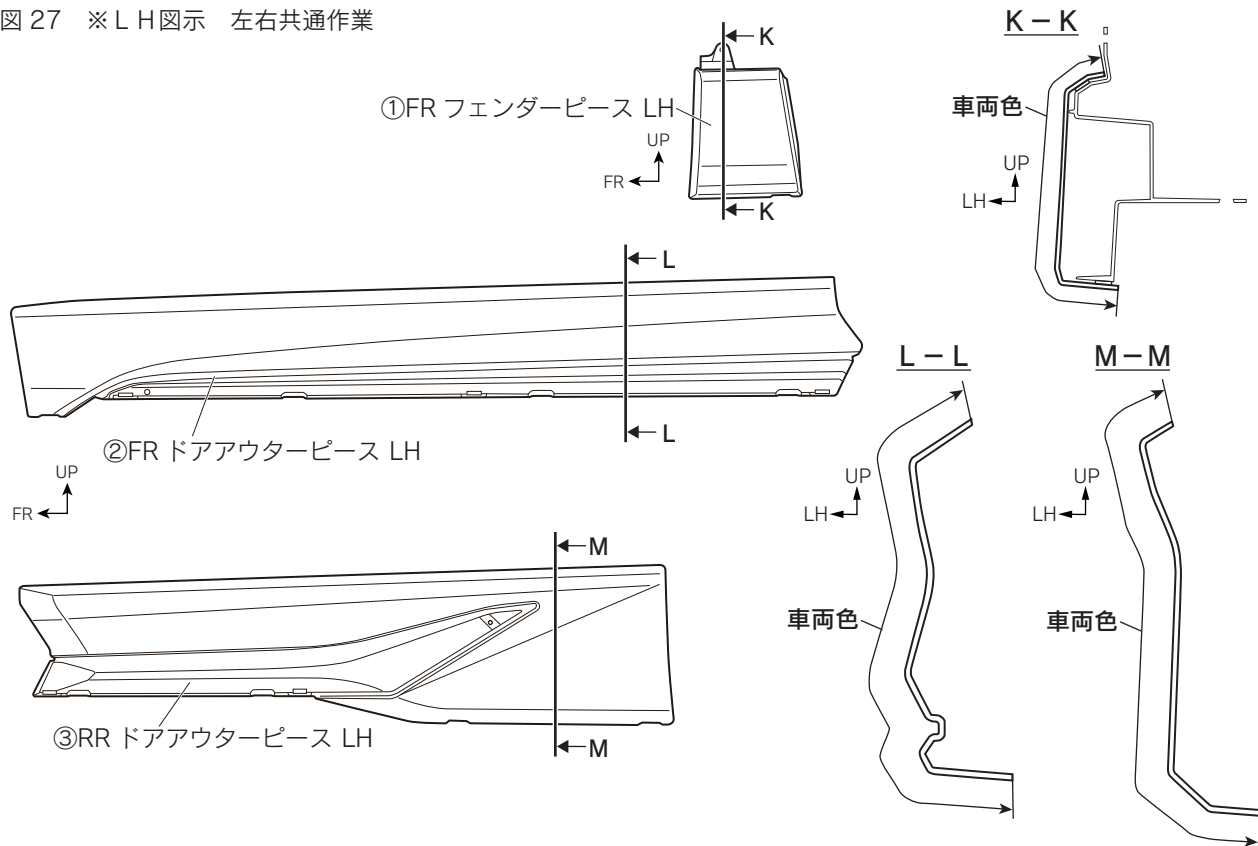
図 27 ※LH図示 左右共通作業
