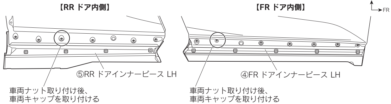
図 11 ※LH図示 左右共通作業
