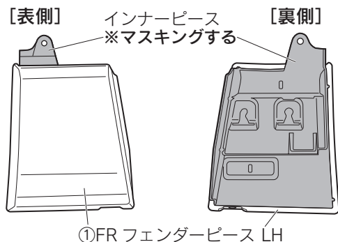
図 26 ※LH図示 左右共通作業
