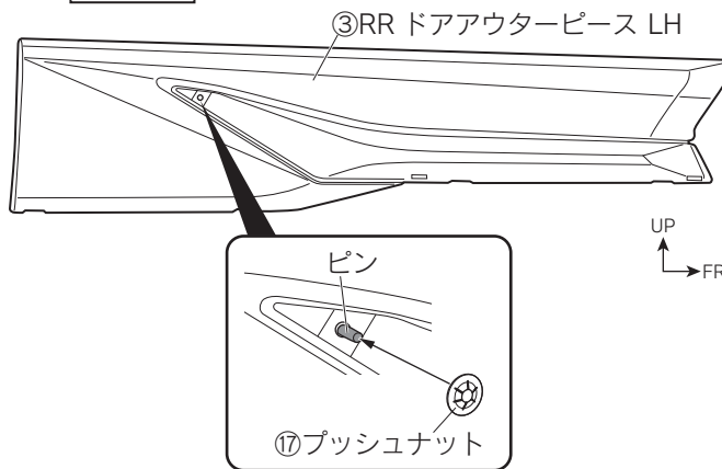
図 37 裏面視 ※LH図示 左右共通作業
