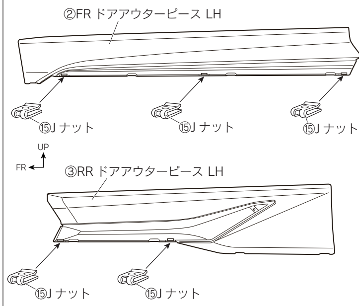
図 30 ※ L H 図示 左右共通作業
