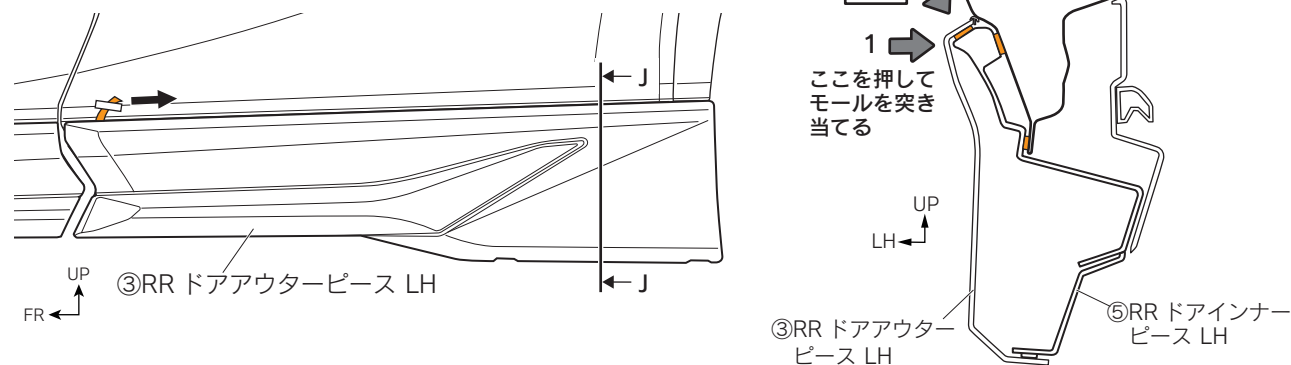
図 25 ※ L H 図示 左右共通作業
