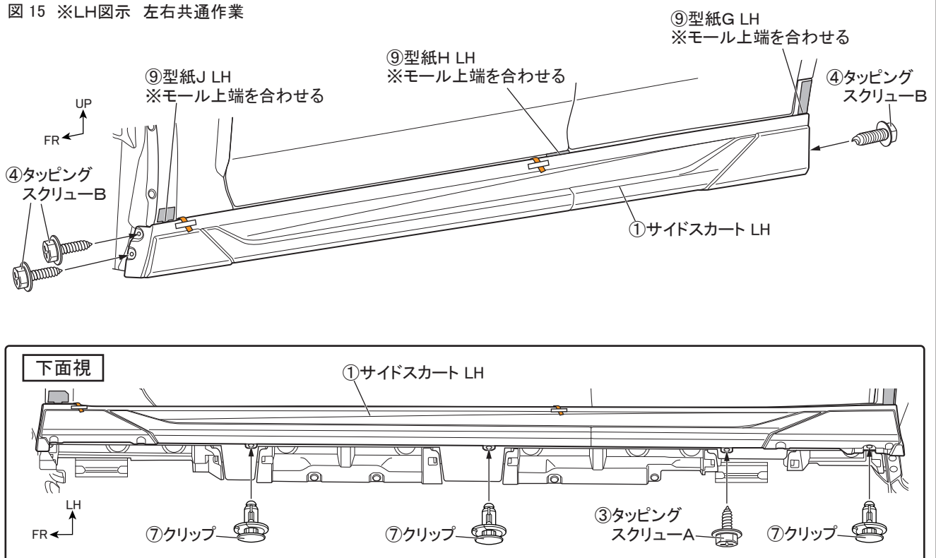
図 15 ※LH図示 左右共通作業
