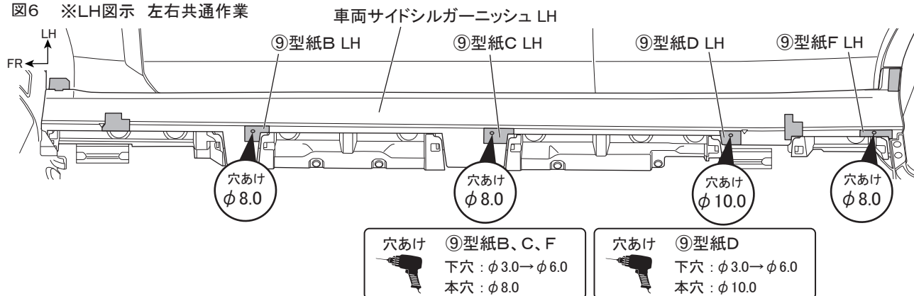
図6 ※LH図示 左右共通作業
