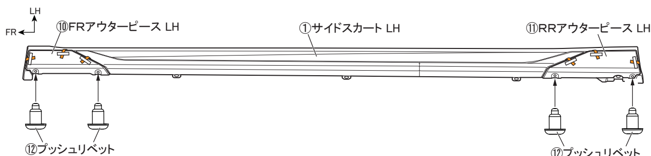
図 23 下面視 ※LH図示 左右共通作業
