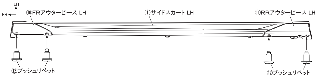
図 18 下面視 ※LH図示 左右共通作業
