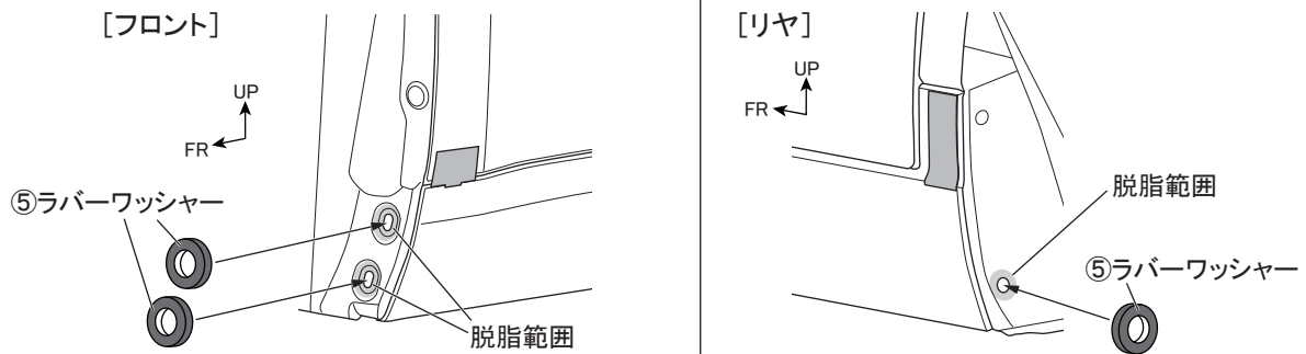
図9 ※LH図示 左右共通作業
