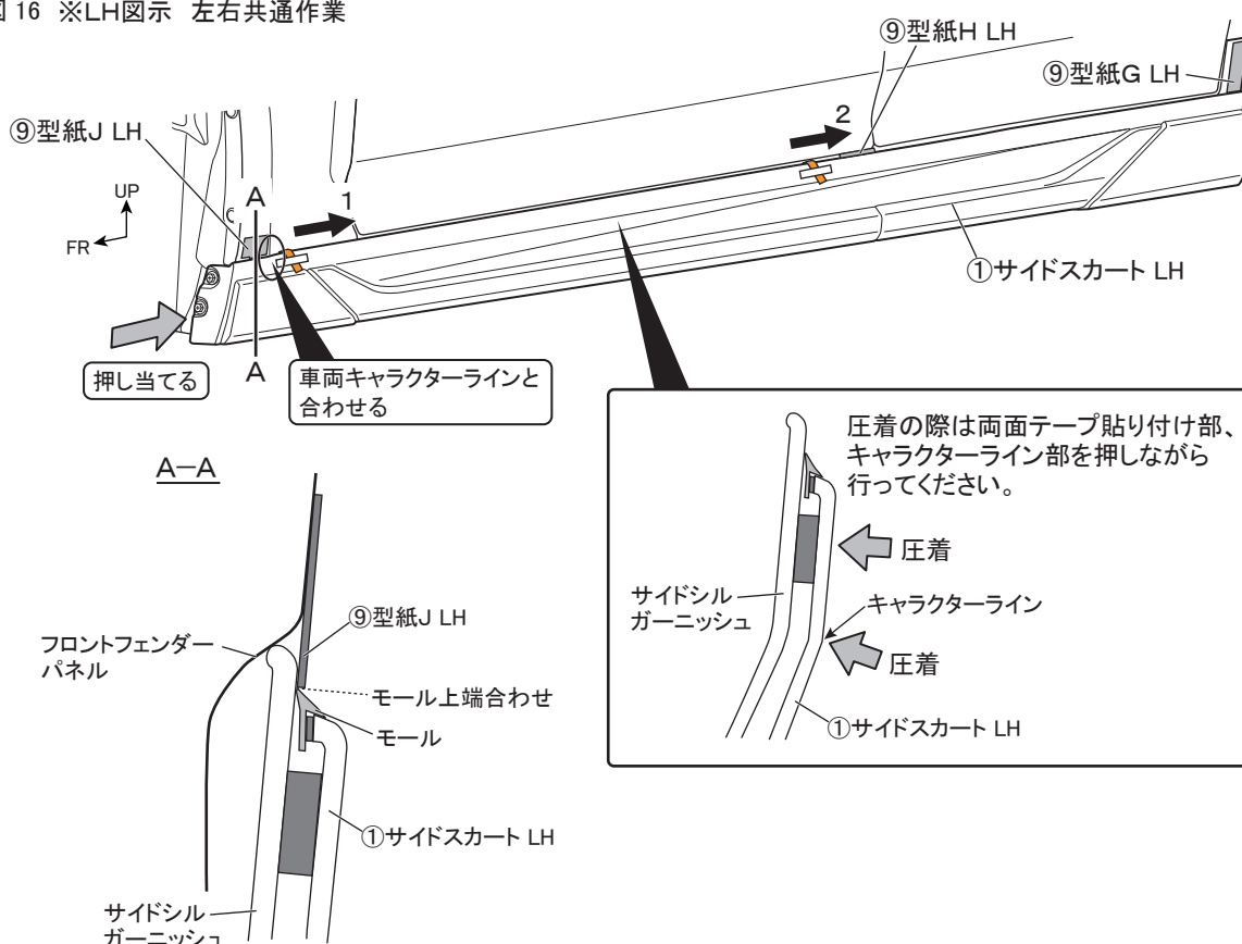
図 16 ※LH図示 左右共通作業
