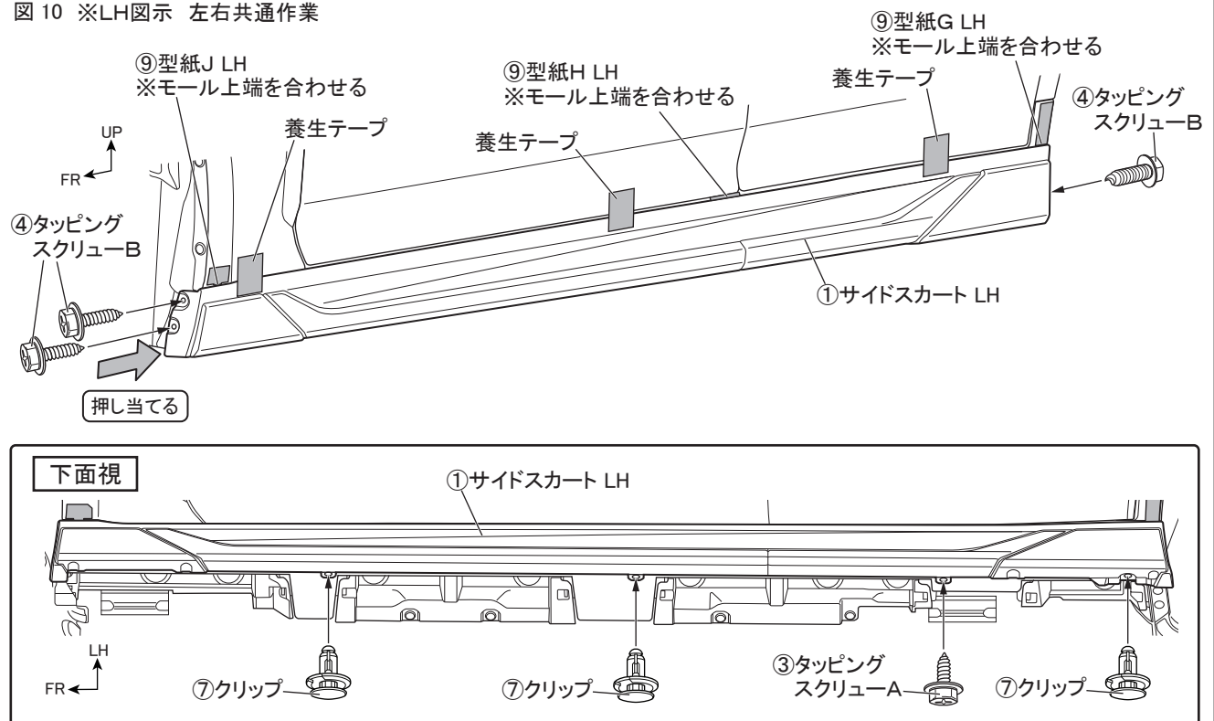
図10 ※LH図示 左右共通作業
