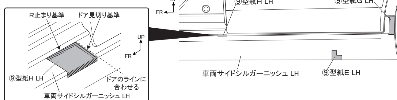
図5 ※LH図示 左右共通作業
