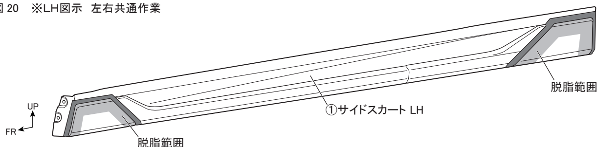
図 20 ※LH図示 左右共通作業
