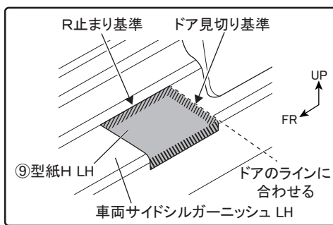
図5 ※LH図示 左右共通作業
