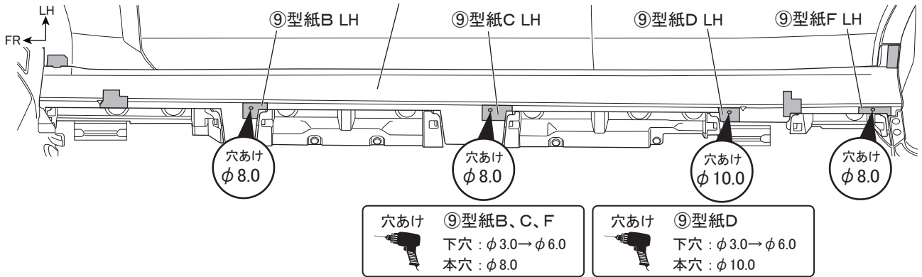
図6 ※LH図示 左右共通作業
