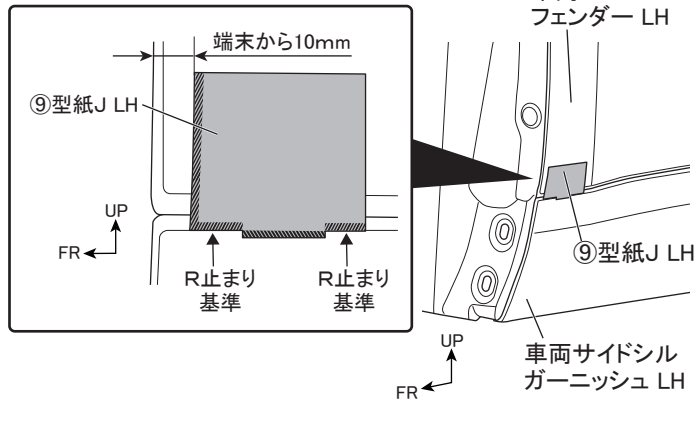
図4 ※LH図示 左右共通作業
