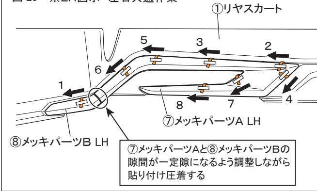
図 29 ※LH図示 左右共通作業
