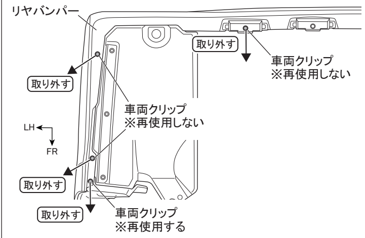
図1 下面視 ※LH図示 左右共通作業
