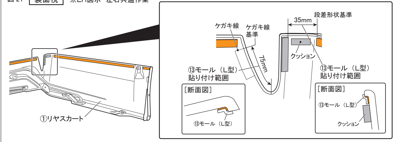
図 21 裏面視 ※LH図示 左右共通作業
