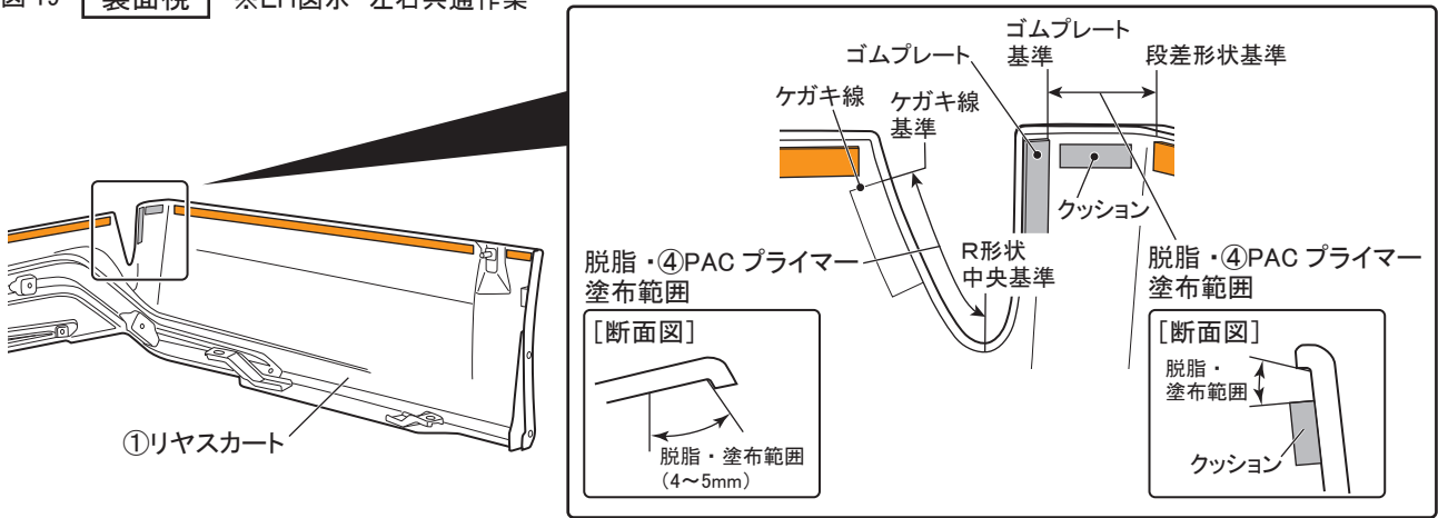
図 19 裏面視 ※LH図示 左右共通作業
