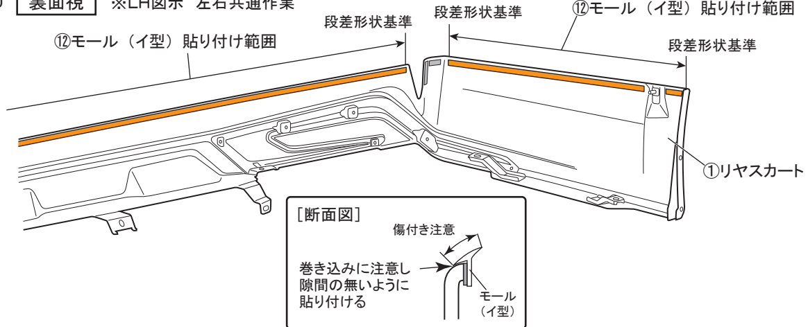
図 20 裏面視 ※LH図示 左右共通作業
