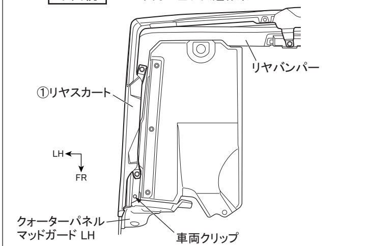
図 14 下面視 ※LH図示 左右共通作業
