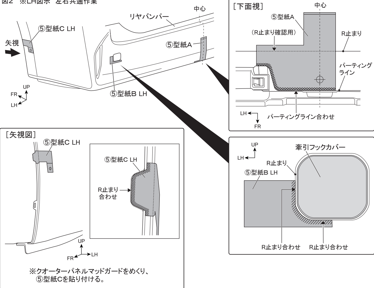
図2 ※LH図示 左右共通作業
