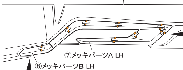
図 28 ※LH図示 左右共通作業
