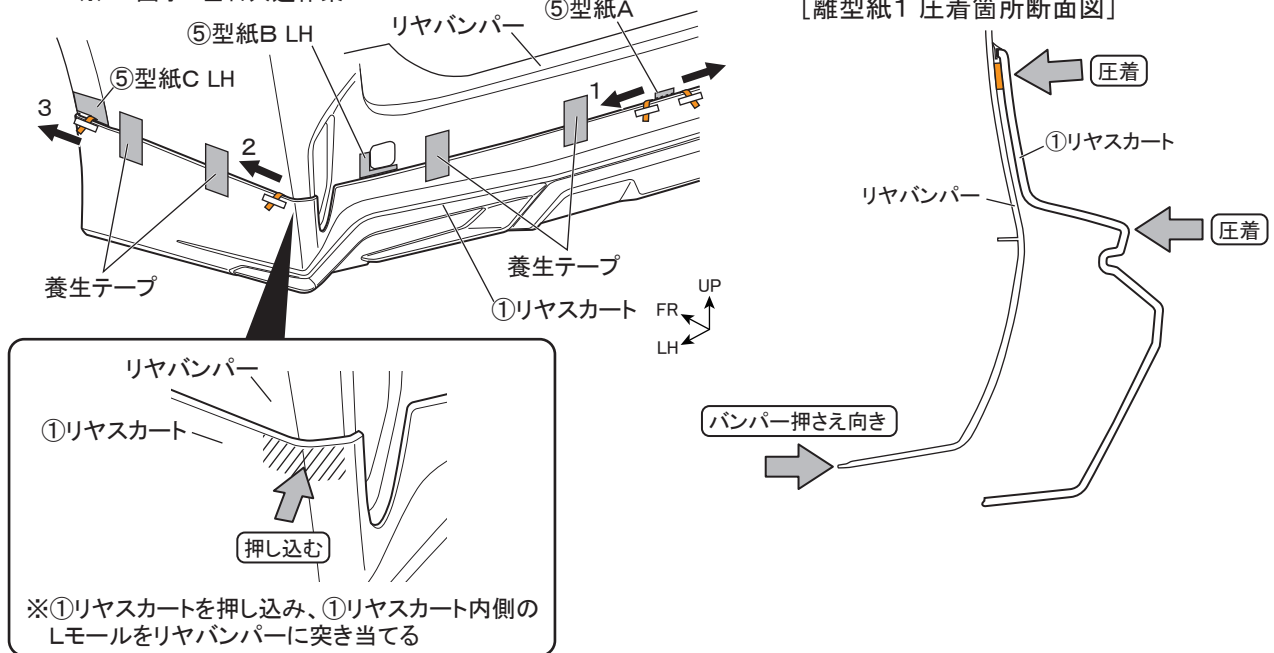
図 13 ※LH図示 左右共通作業
