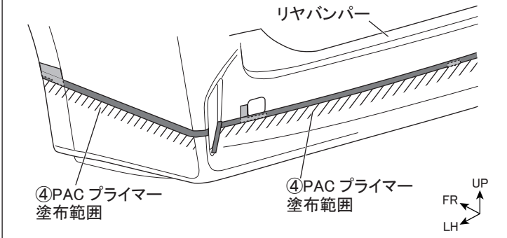
図 10 ※LH図示 左右共通作業
