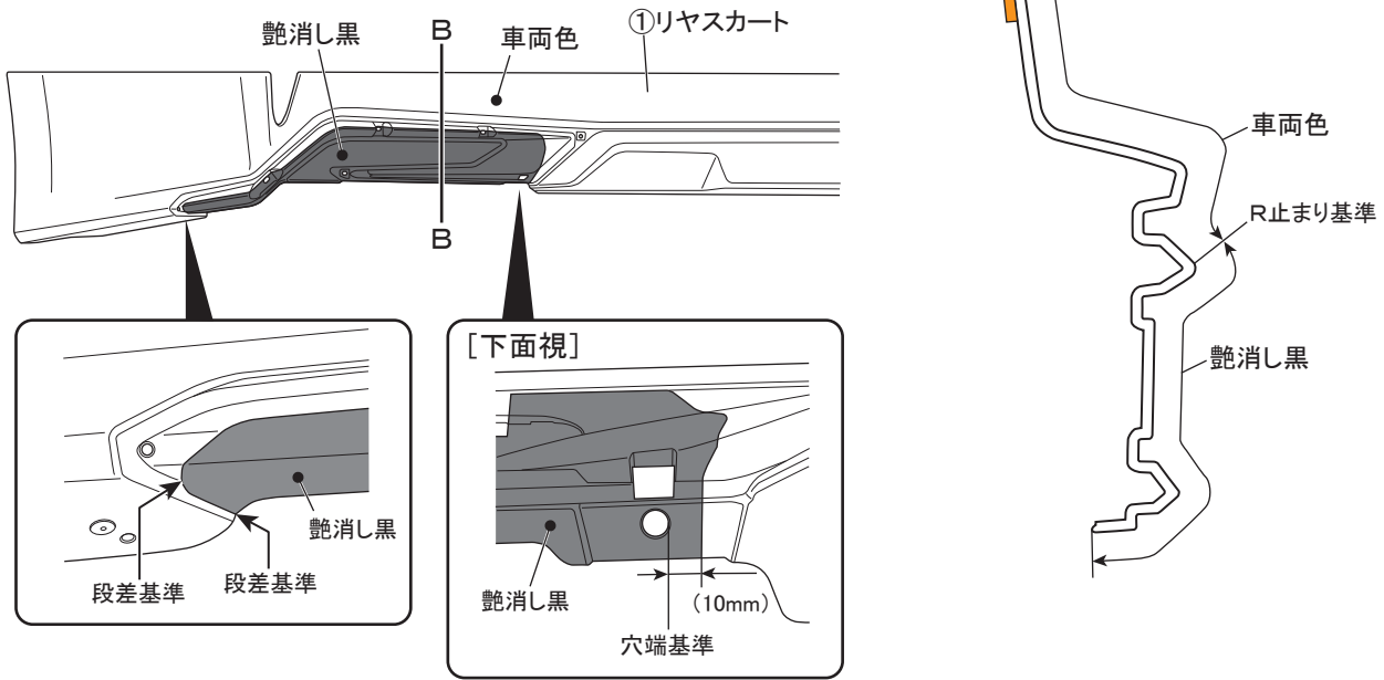
図 17 ※LH図示 左右共通作業
