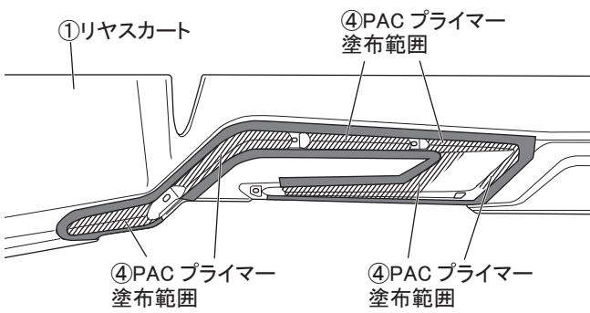
図 25 ※LH図示 左右共通作業
