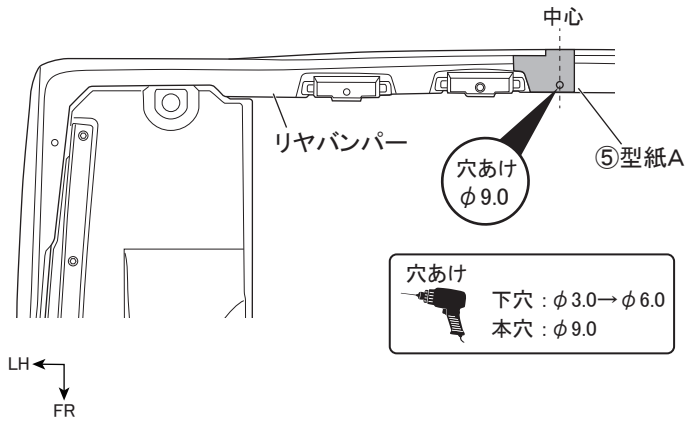
図3 下面視 ※LH図示 左右共通作業
