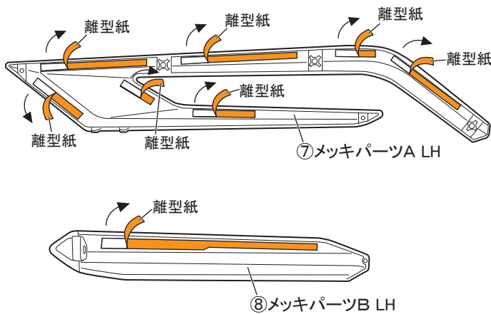
図 27 裏面視 ※LH図示 左右共通作業
