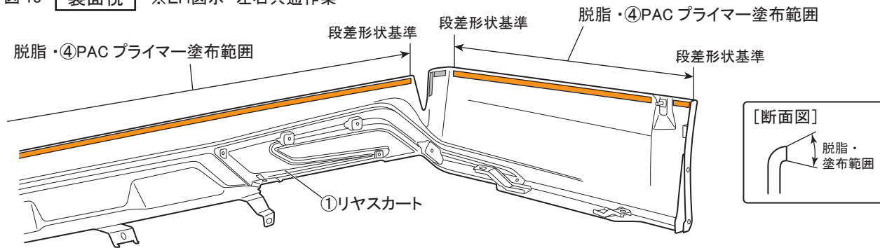
図 18 裏面視 ※LH図示 左右共通作業
