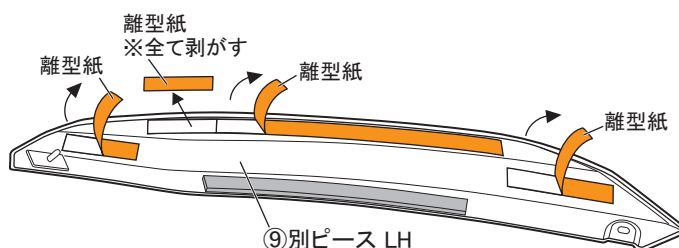
図 24 裏面視 ※LH図示 左右共通作業
