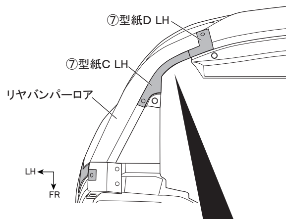
下面視 [⑦型紙Cを貼り付ける]
