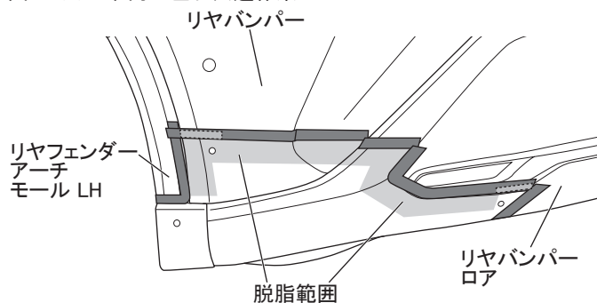
図 10 ※LH図示 左右共通作業
