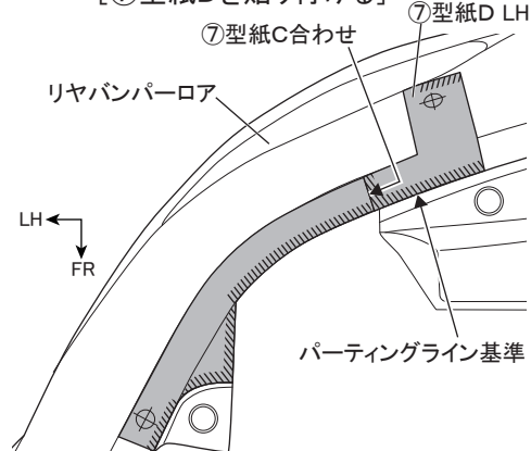
[⑦型紙Dを貼り付ける]
