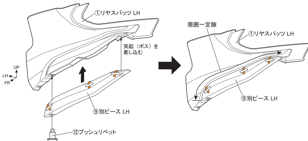
図 25 ※LH図示 左右共通作業
