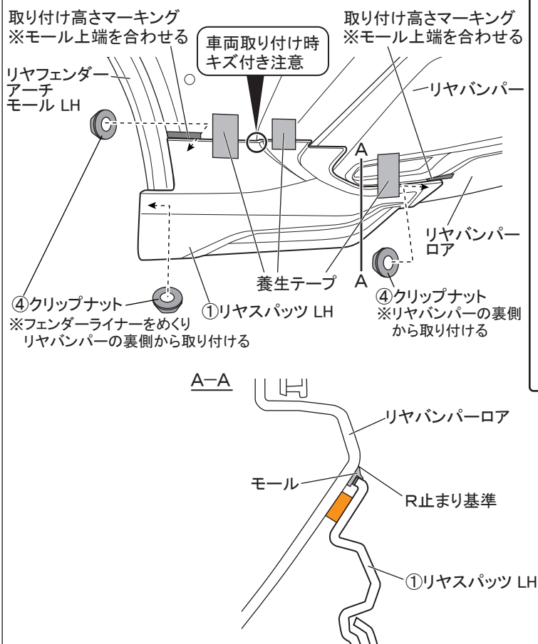
図8 ※LH図示 左右共通作業
