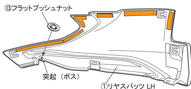
図 27 裏面視 ※LH図示 左右共通作業
