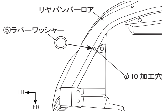
図6 下面視 ※LH図示 左右共通作業
