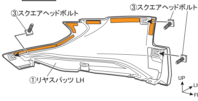
図7 裏面視 ※LH図示 左右共通作業
