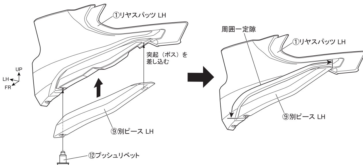
図 20 ※LH図示 左右共通作業
