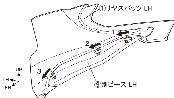
図 26 ※LH図示 左右共通作業
