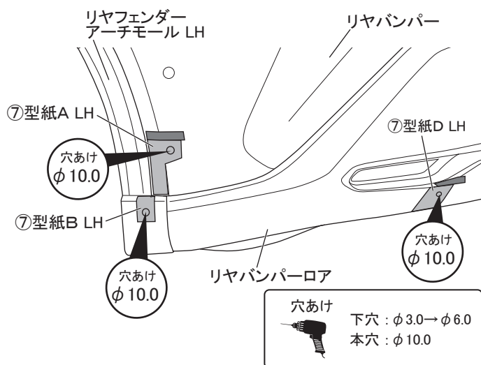
図5 ※LH図示 左右共通作業
