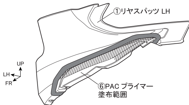
図 23 ※LH図示 左右共通作業
