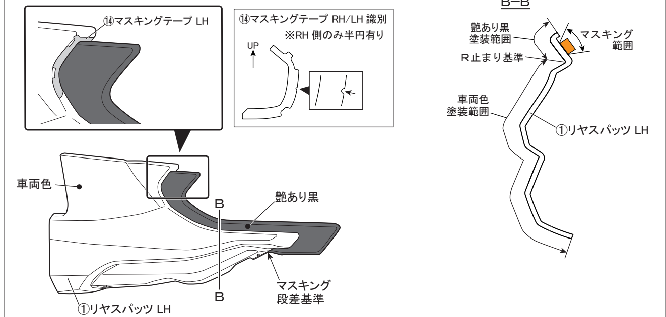
図 17 ※LH図示 左右共通作業
