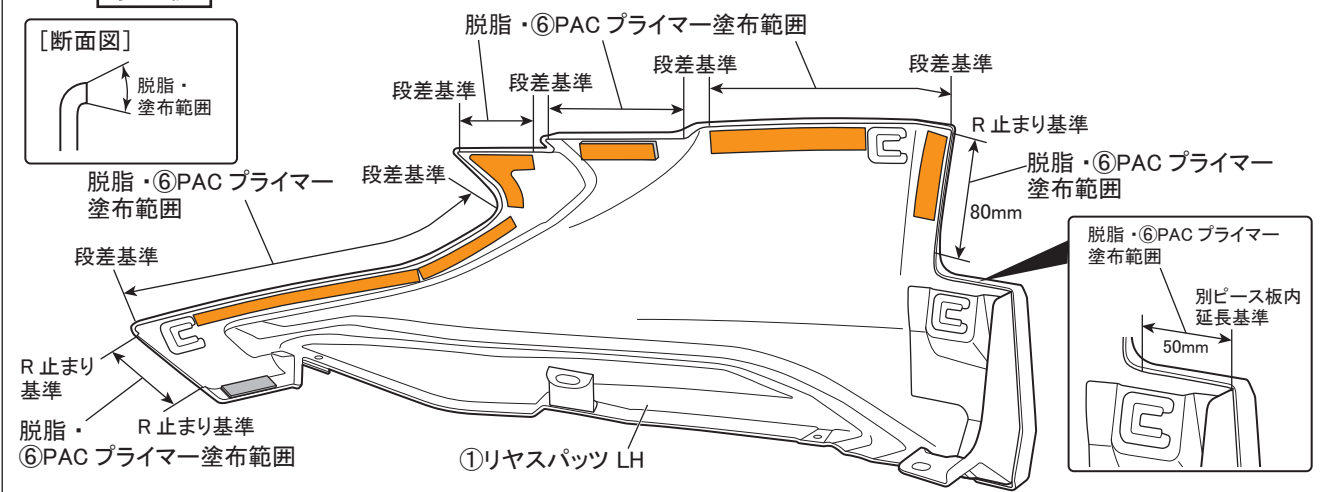
図 18 裏面視 ※LH図示 左右共通作業
