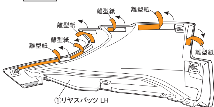
図 12 裏面視 ※LH図示 左右共通作業
