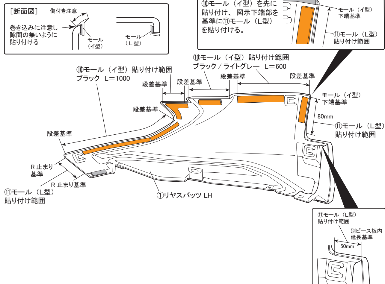
図 19 裏面視 ※LH図示 左右共通作業
