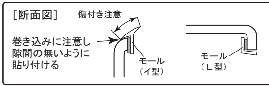
図 19 裏面視 ※LH図示 左右共通作業
