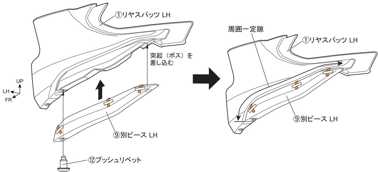
図 25 ※LH図示 左右共通作業
