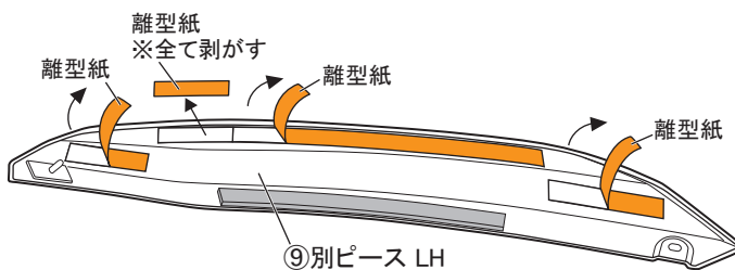
図 24 裏面視 ※LH図示 左右共通作業
