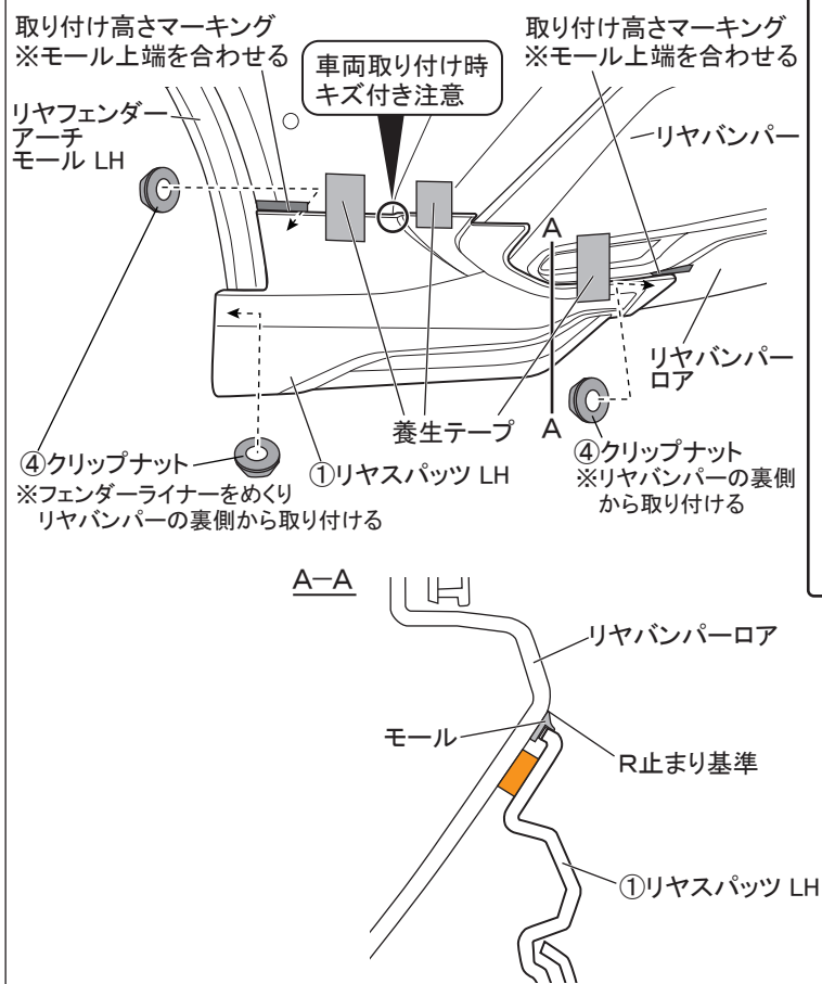
図8 ※LH図示 左右共通作業
