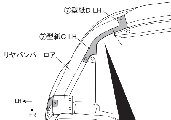
図3 下面視 ※LH図示 左右共通作業
