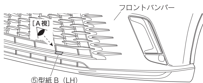
図4 ※LH図示 左右共通作業
