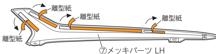
図 22 裏面視 ※ LH 図示 左右共通作業
