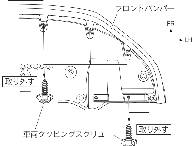
図1 下面視 ※LH図示 左右共通作業
