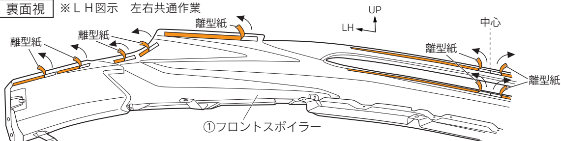
図9 裏面視 ※LH図示 左右共通作業
