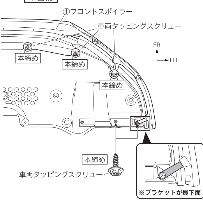
図 12 下面視 ※ L H 図示 左右共通作業
