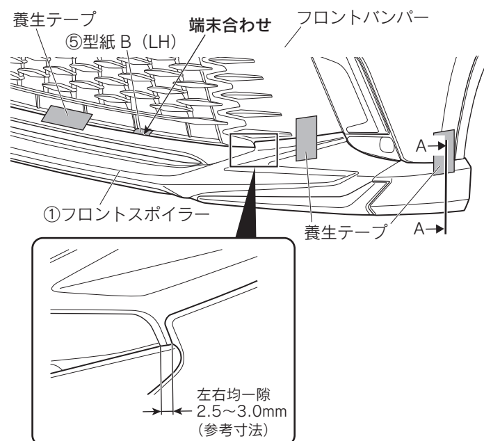
図5 ※LH図示 左右共通作業
