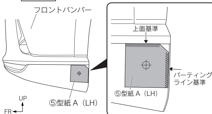
図2 側面視 ※LH図示 左右共通作業
