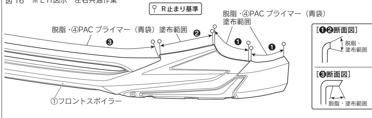
図 16 ※L H図示 左右共通作業
