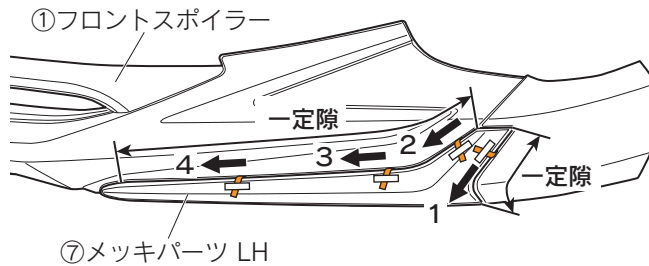
図 24 ※LH図示 左右共通作業
