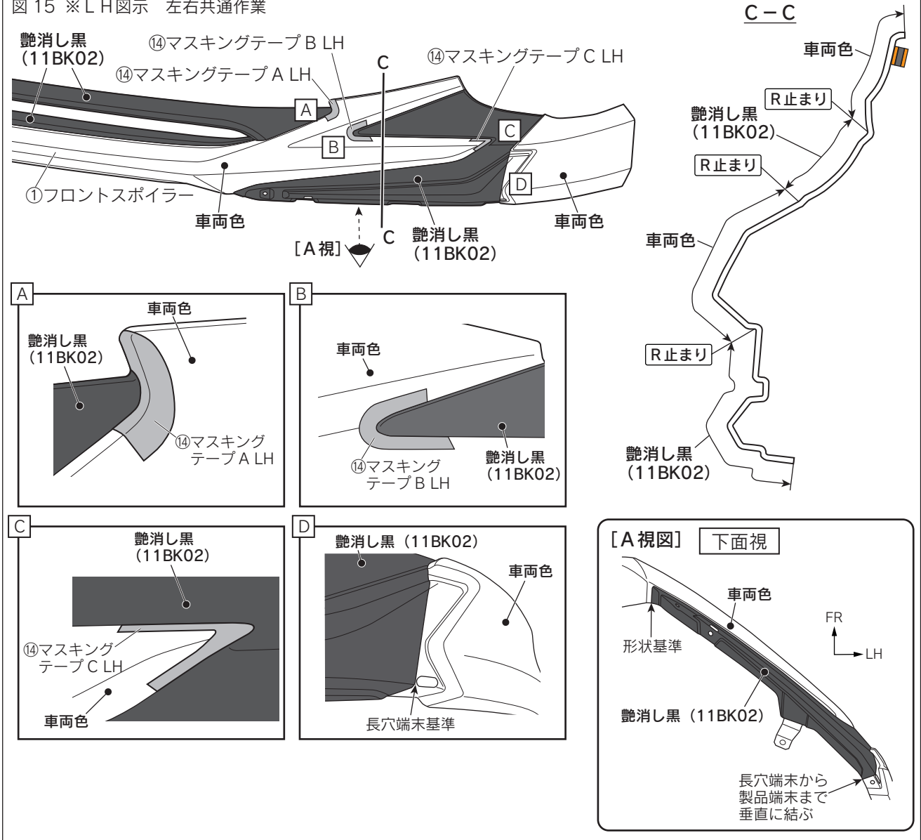
図 15 ※LH図示 左右共通作業
