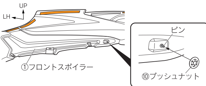
図 25 裏面視 ※LH図示 左右共通作業
