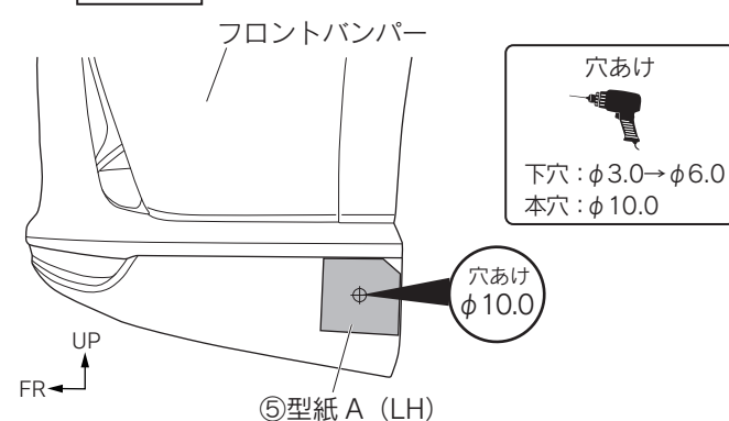
図3 側面視 ※LH図示 左右共通作業
