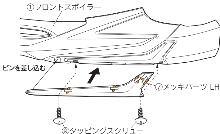
図 23 ※ LH 図示 左右共通作業
