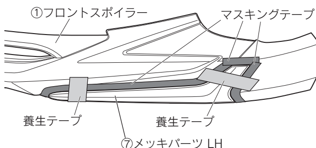
図 19 ※LH図示 左右共通作業
