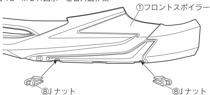
図 18 ※LH図示 左右共通作業
