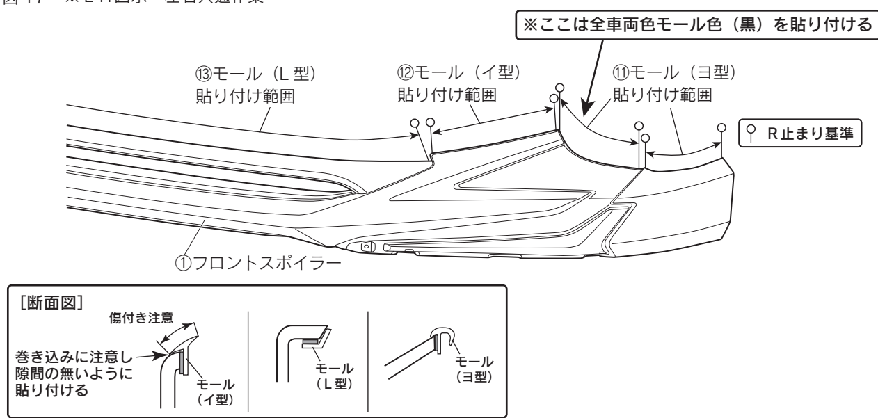
図 17 ※L H図示 左右共通作業
