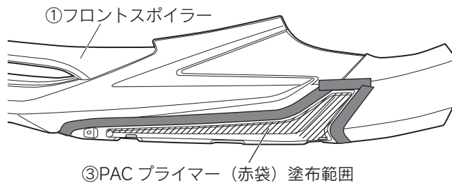
図 21 ※ LH 図示 左右共通作業
