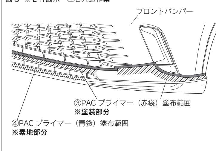
図8 ※LH図示 左右共通作業
