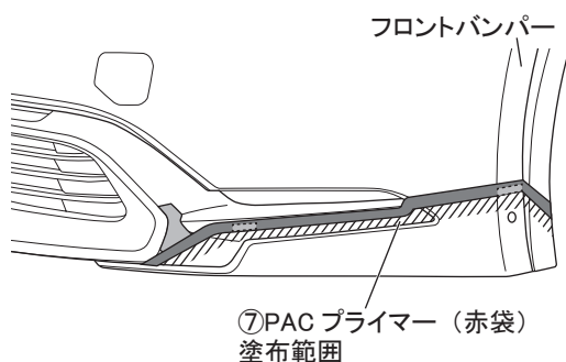
図 11 ※LH図示 左右共通作業
