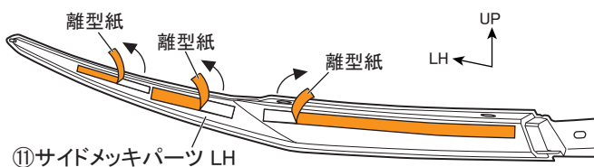
図 25 裏面視 ※LH図示 左右共通作業
