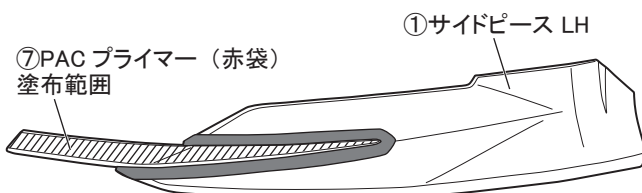
図 24 ※LH図示 左右共通作業
