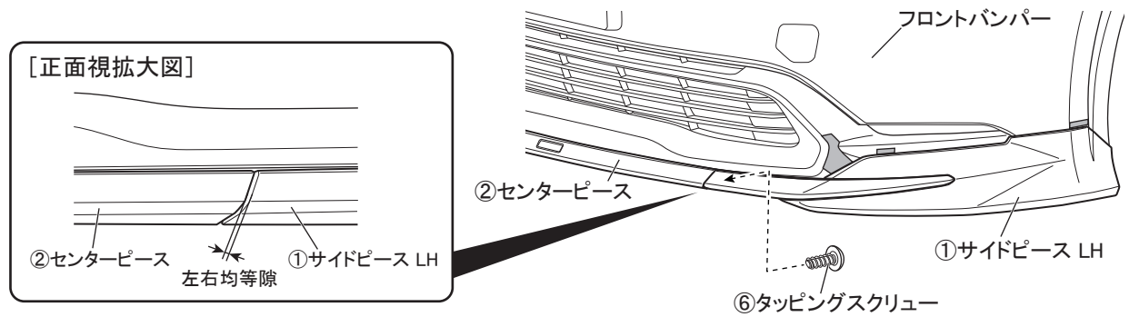
図 16 ※LH図示 左右共通作業
