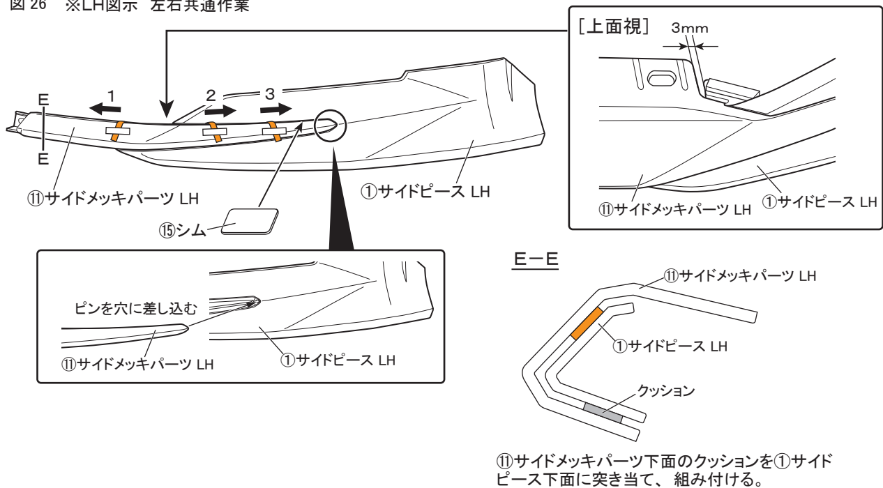
図 26 ※LH図示 左右共通作業
