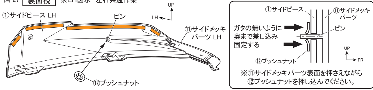
図 27 裏面視 ※LH図示 左右共通作業
