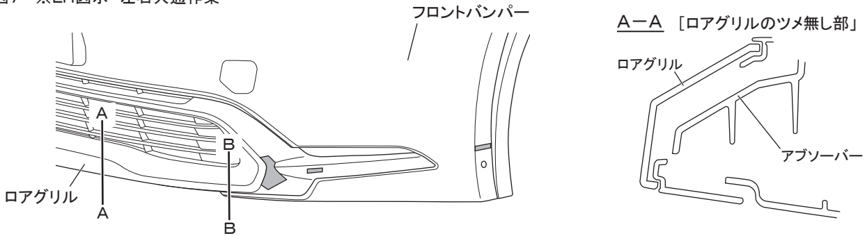
図7 ※LH図示 左右共通作業
