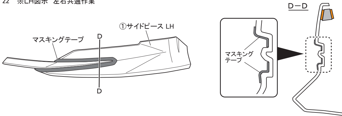
図 22 ※LH図示 左右共通作業
