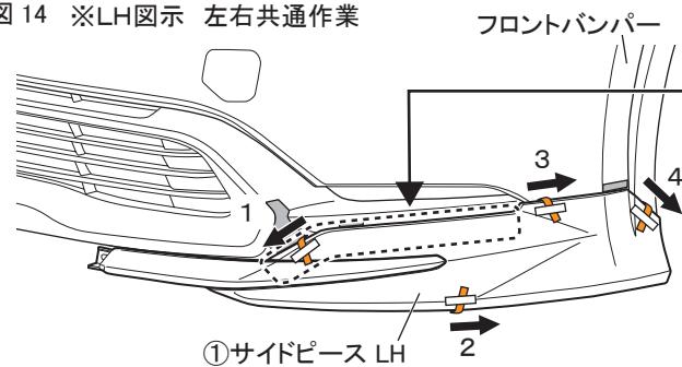
図 14 ※LH図示 左右共通作業
