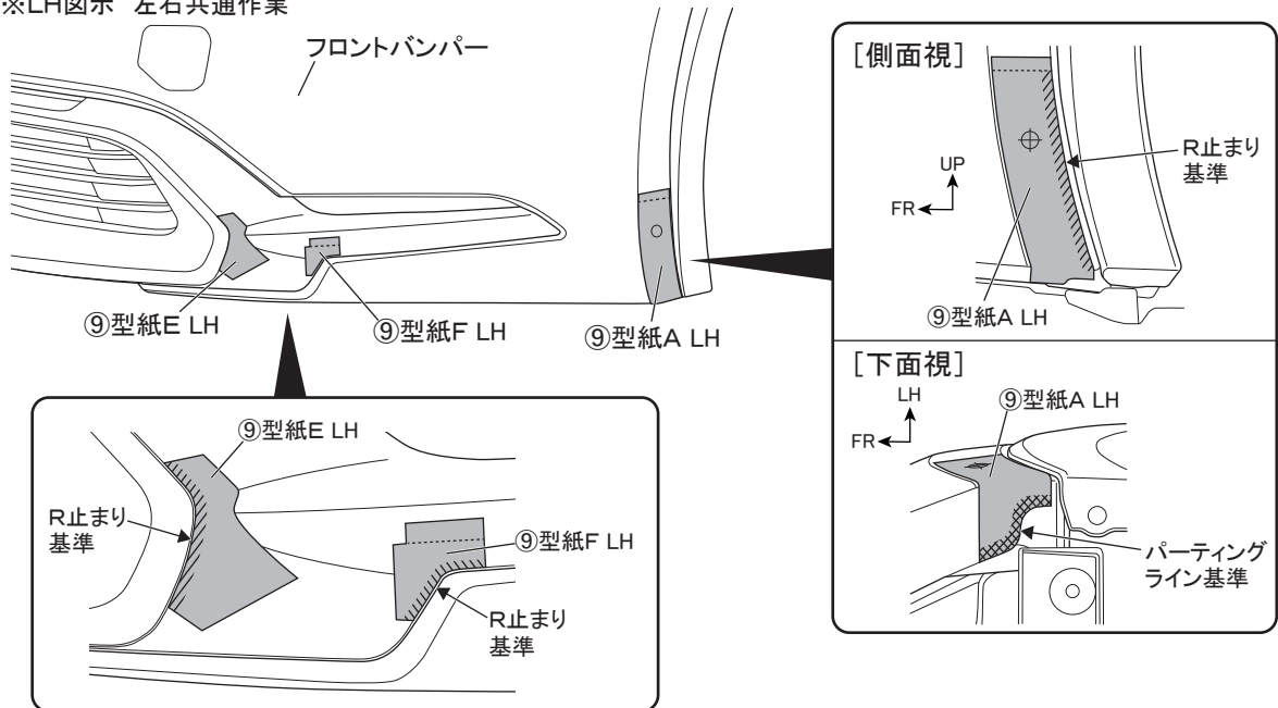
図2 ※LH図示 左右共通作業
