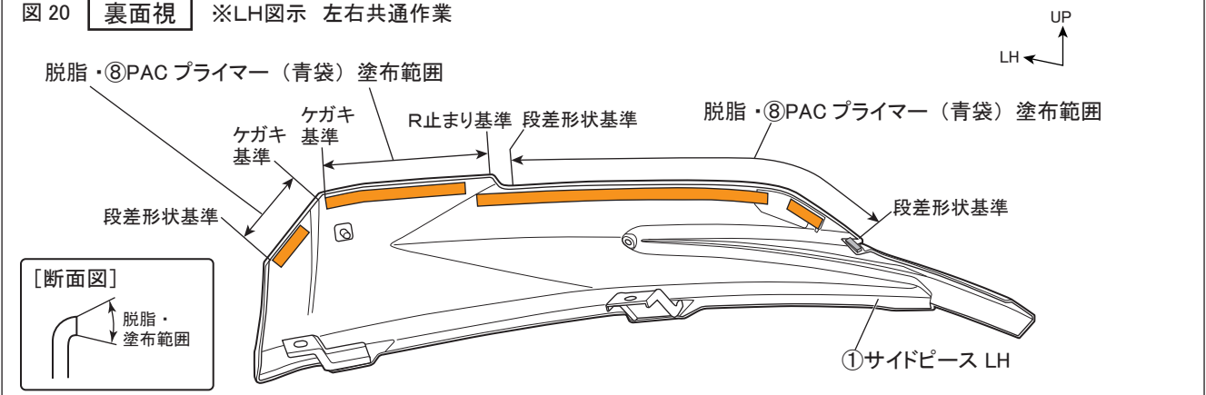
図 20 裏面視 ※LH図示 左右共通作業
