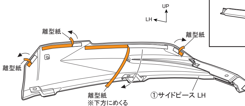
図 12 裏面視 ※LH図示 左右共通作業
