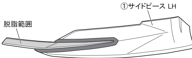
図 23 ※LH図示 左右共通作業
