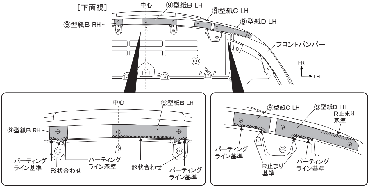
図3 ※LH図示 左右共通作業
