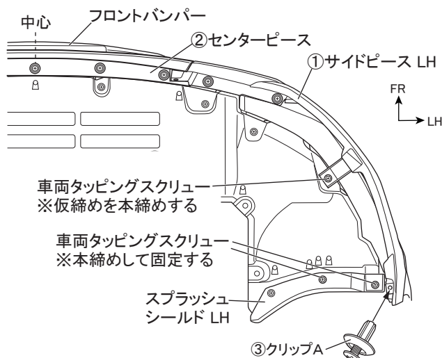
図 17 下面視 ※LH図示 左右共通作業
