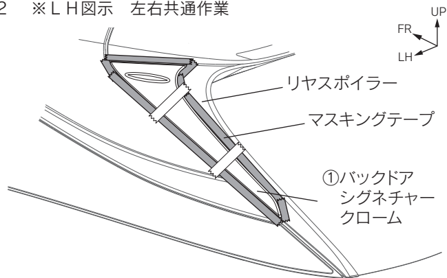
図2 ※LH図示 左右共通作業
