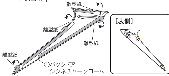
図5 裏面視 ※LH図示 左右共通作業
