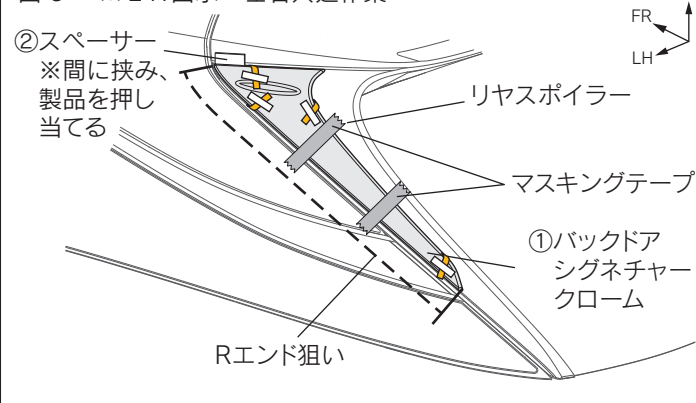
図6 ※LH図示 左右共通作業
