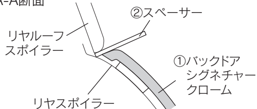
A-A断面
