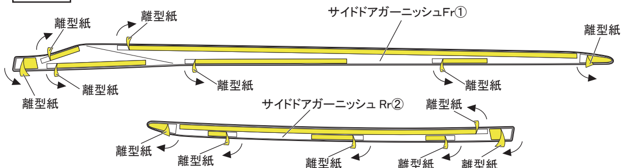
図5 裏面視 ※LH図示 左右共通作業
