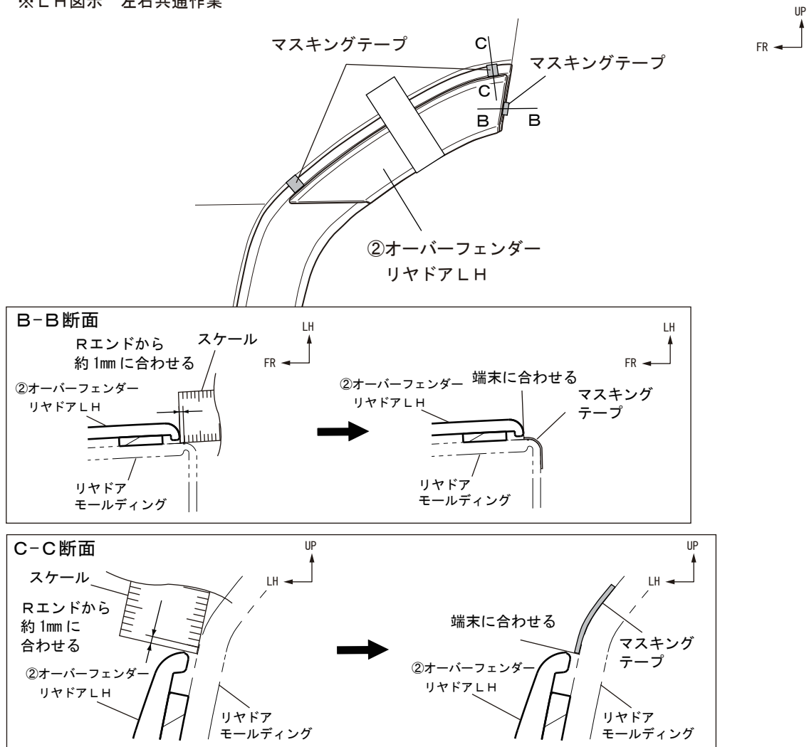
図7 ※LH図示 左右共通作業
