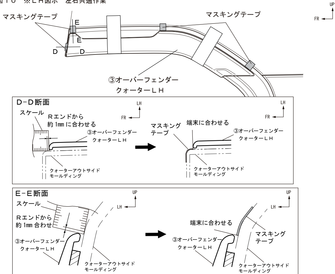
図10 ※LH図示 左右共通作業
