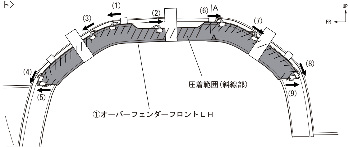
図15 ※LH図示 左右共通作業
