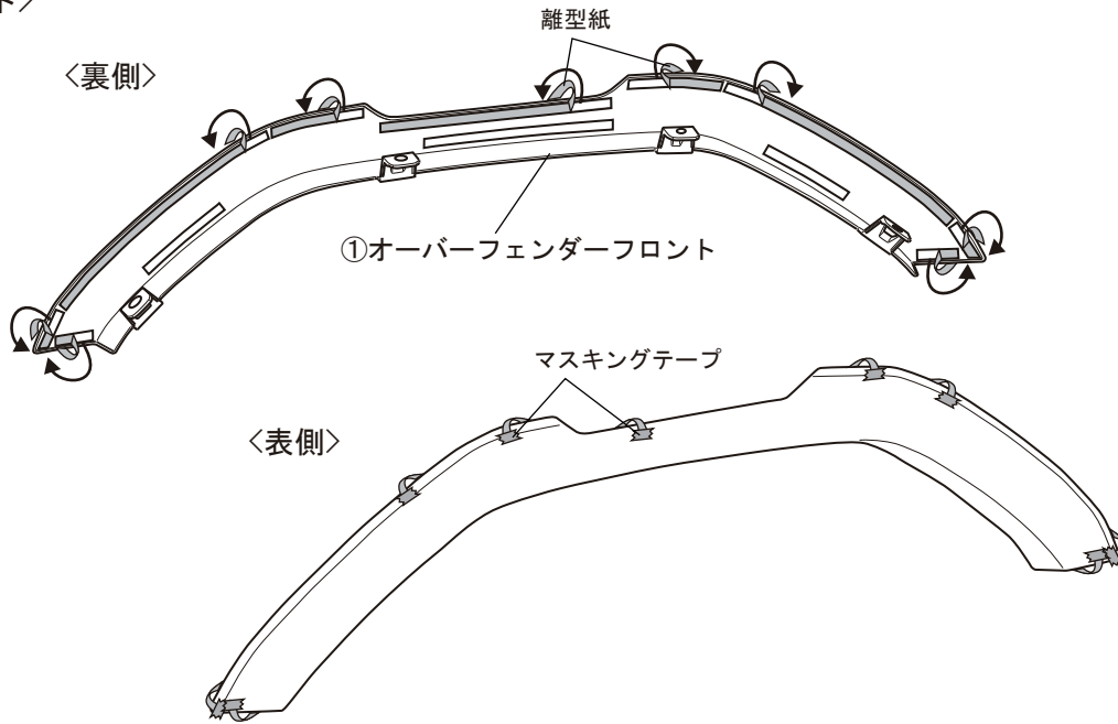
図13 ※LH図示 左右共通作業 〈フロント〉
