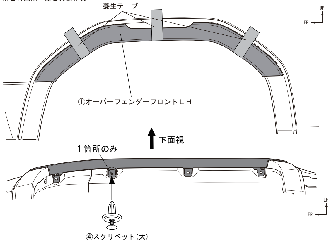
図2 ※LH図示 左右共通作業
