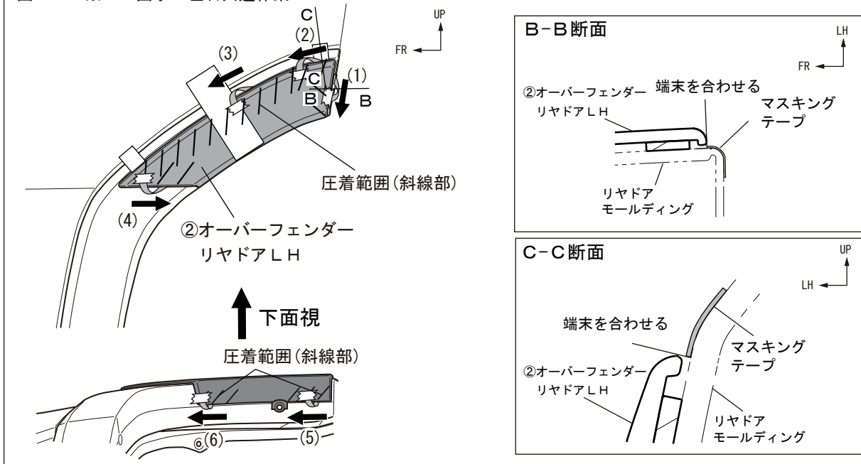
図19 ※LH図示 左右共通作業
