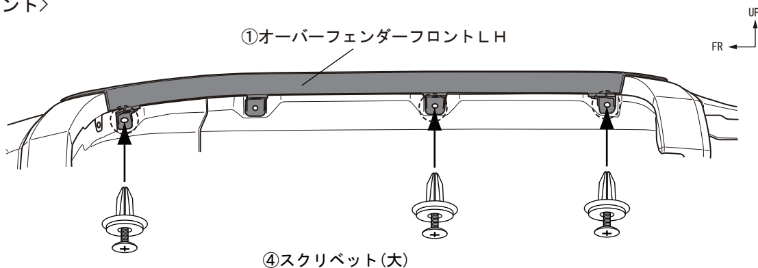
図16 ※LH図示 左右共通作業
