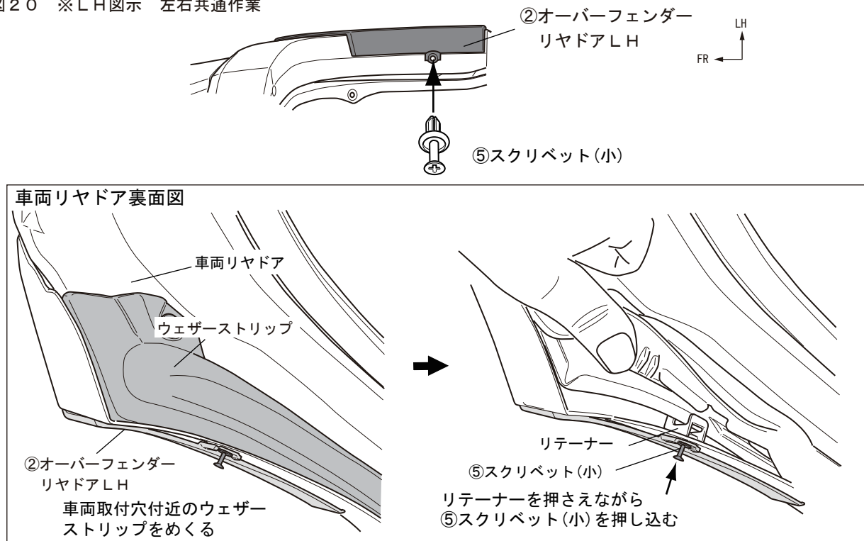
図20 ※LH図示 左右共通作業
