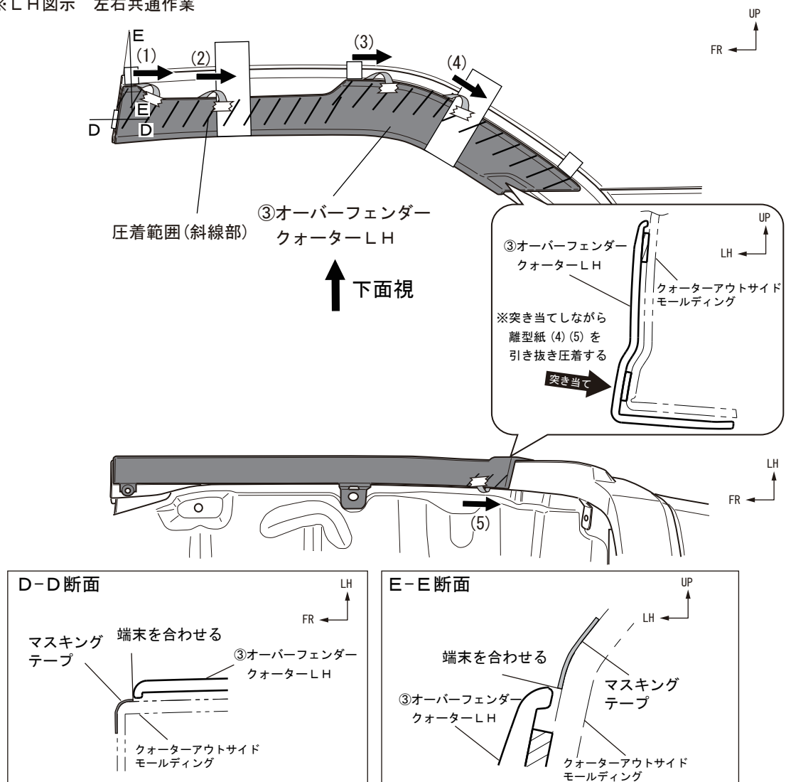
図 2 2 ※LH図示 左右共通作業
