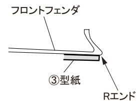
【B-B断面】
