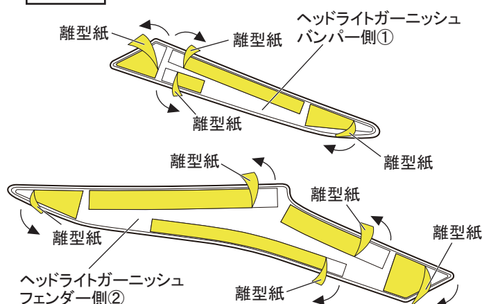
図5 裏面視 ※LH図示 左右共通作業
