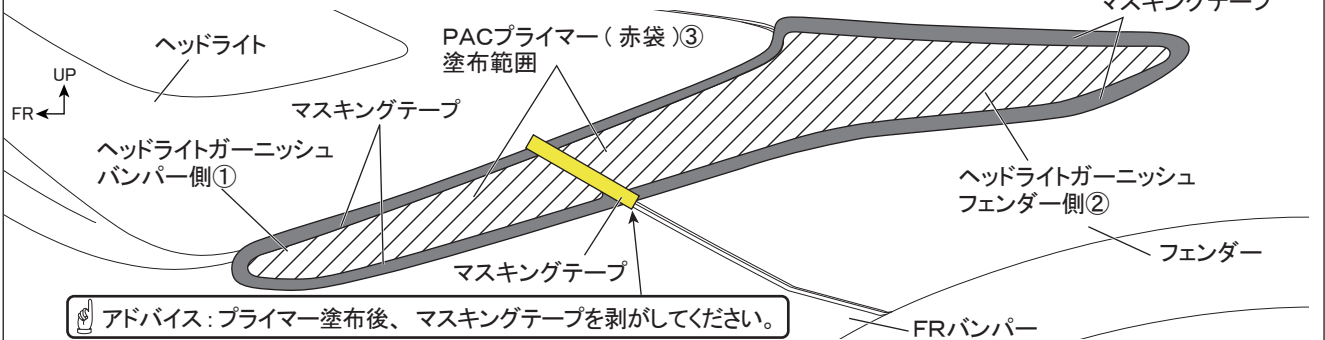
図4 ※LH図示 左右共通作業
