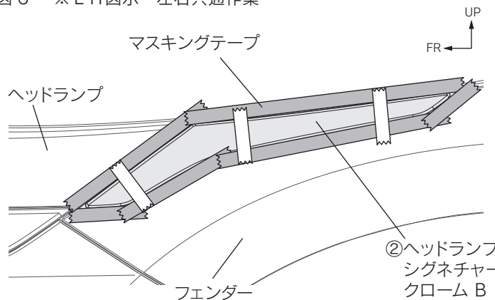
図6 ※LH図示 左右共通作業
