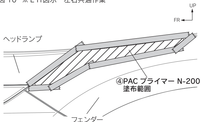
図10 ※LH図示 左右共通作業
