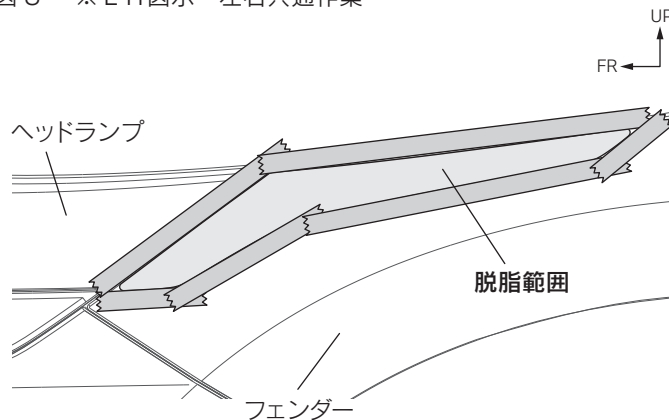
図8 ※LH図示 左右共通作業
