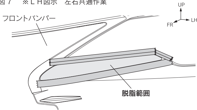
図7 ※LH図示 左右共通作業
