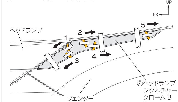
図 15 ※L H図示 左右共通作業
