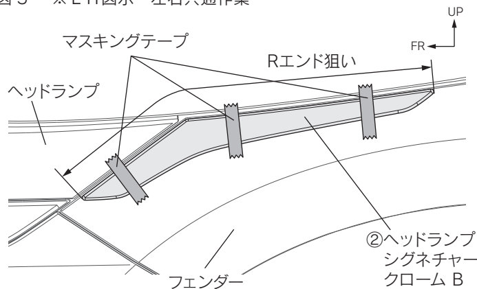
図5 ※LH図示 左右共通作業
