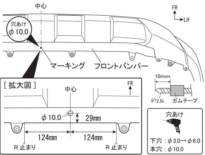
図5 下面視
