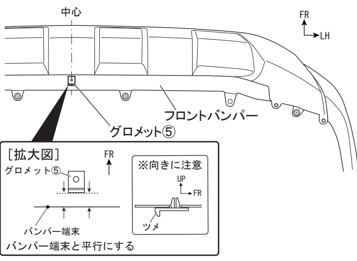
図6 下面視
