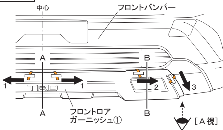
図 13 正面視 ※LH図示 左右共通作業
