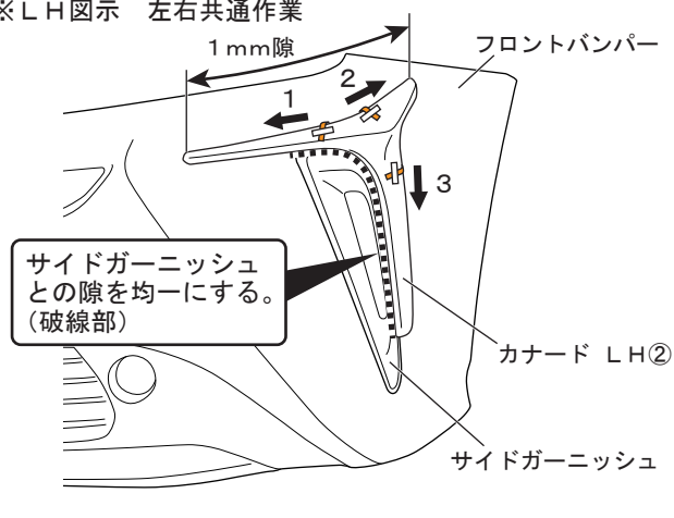
図 10 ※LH図示 左右共通作業
