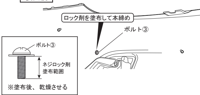
図8 裏面視 ※LH図示 左右共通作業
