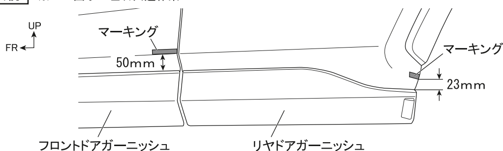
図6 側面視 ※LH図示 左右共通作業
