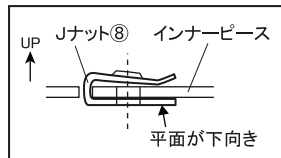
図 17 側面視 ※LH図示 左右共通作業
