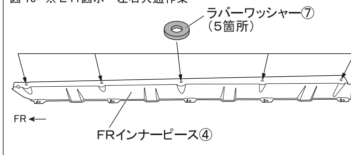
図 13 ※ L H 図示 左右共通作業
