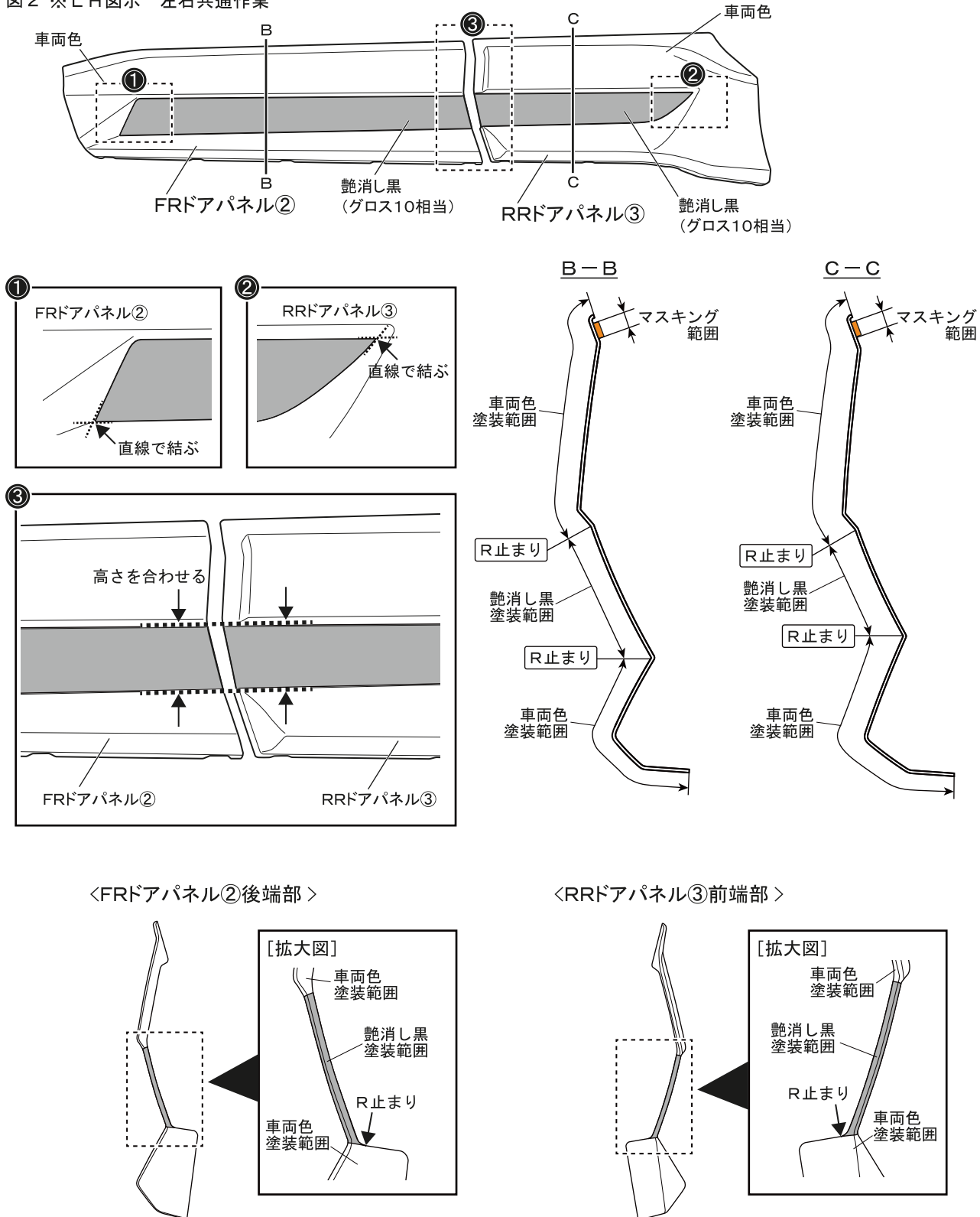
図2 ※LH図示 左右共通作業
