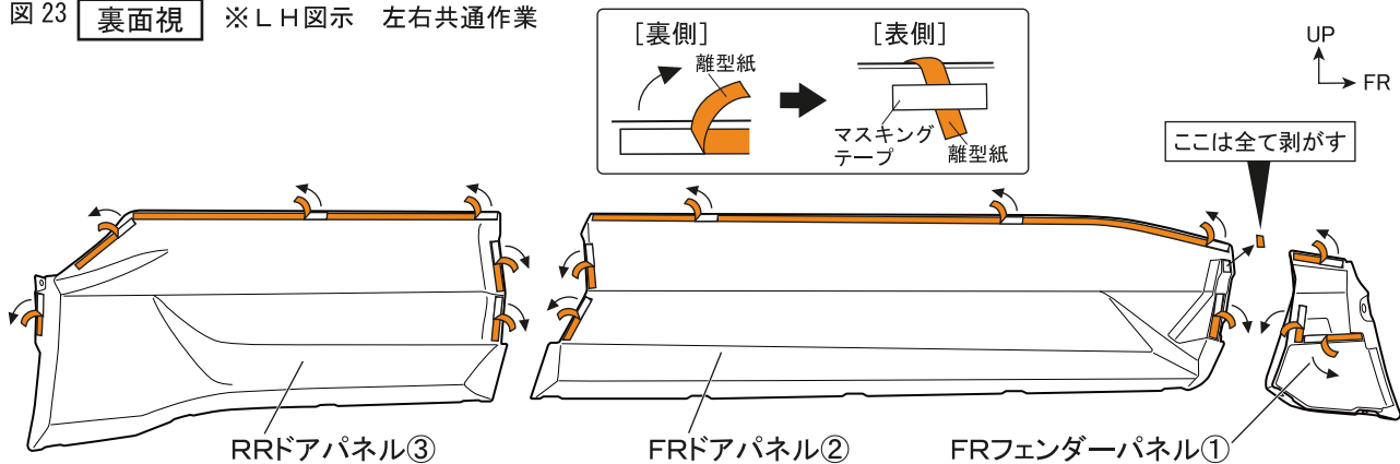
図 23 裏面視 ※L H図示 左右共通作業
