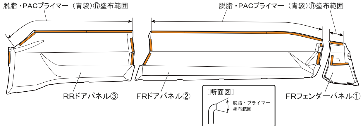
図3 裏面視 ※LH図示 左右共通作業
