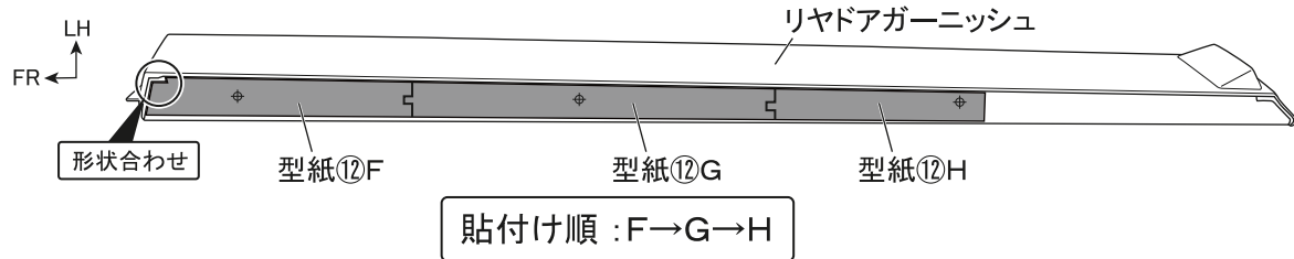
図9 下面視 ※LH図示 左右共通作業
