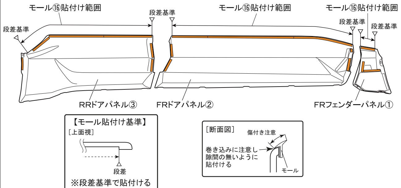
図4 裏面視 ※LH図示 左右共通作業
