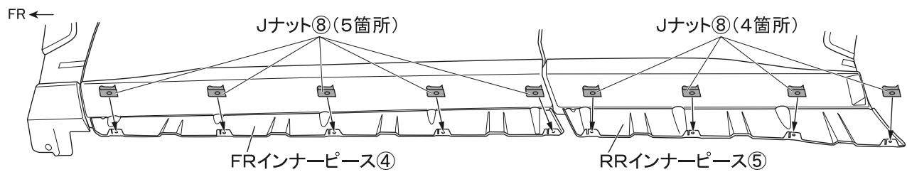
図 16 ※LH図示 左右共通作業
