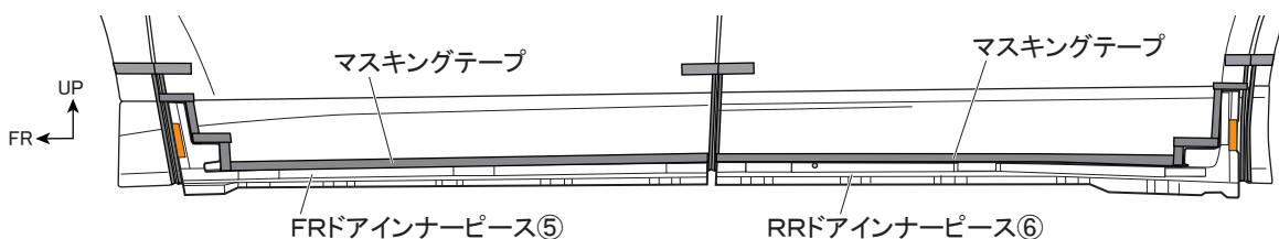
図8 ※LH図示 左右共通作業
