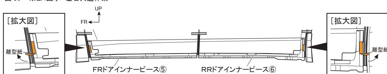
図 30 ※LH図示 左右共通作業
