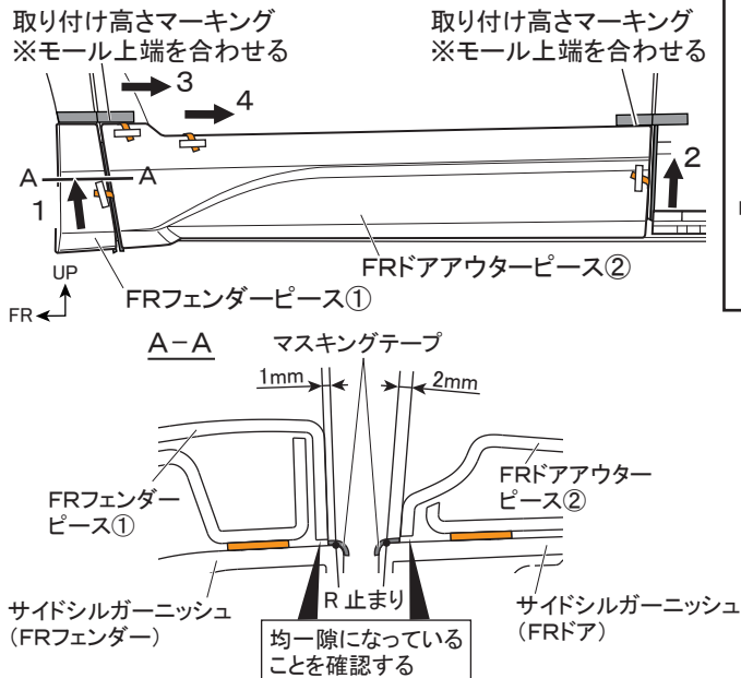
図 31 ※LH図示 左右共通作業
