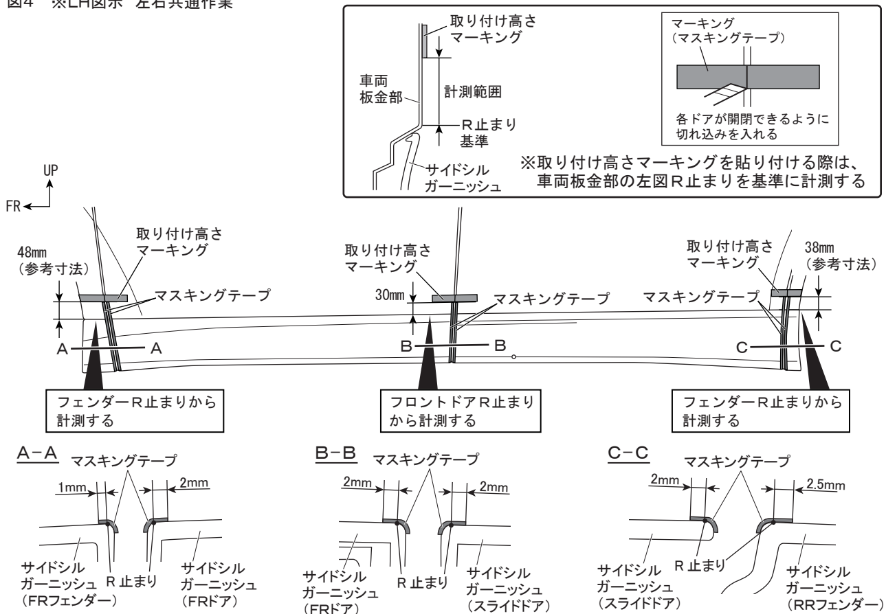
図4 ※LH図示 左右共通作業
