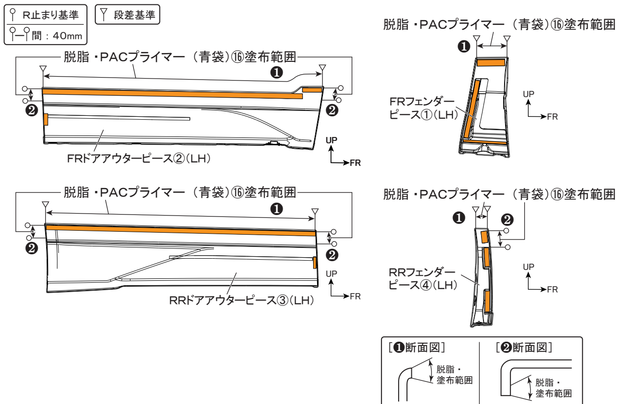
図 34 裏面視 ※LH図示 左右共通作業
