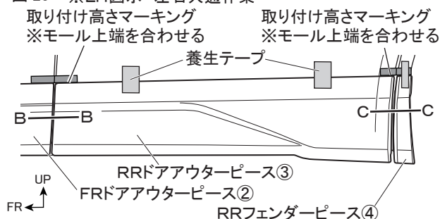
図 20 ※LH図示 左右共通作業
