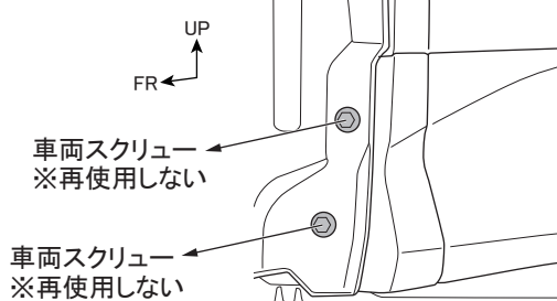
図5 ※LH図示 左右共通作業
