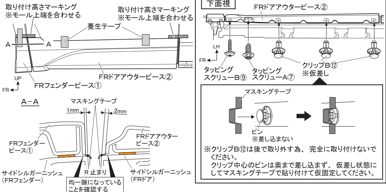
図 19 ※LH図示 左右共通作業
