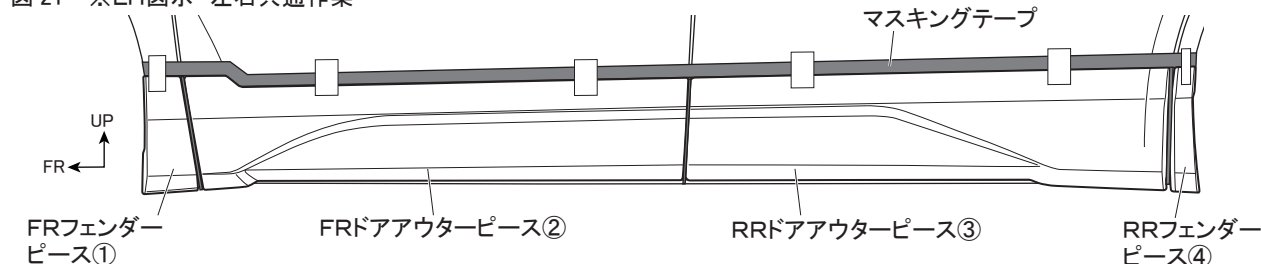
図 21 ※LH図示 左右共通作業
