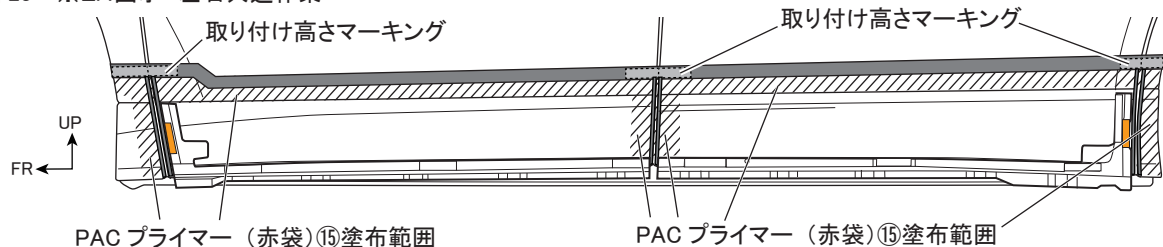
図 23 ※LH図示 左右共通作業
