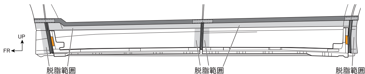
図 22 ※LH図示 左右共通作業
