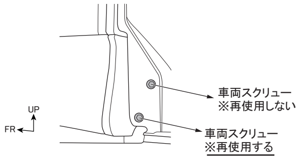
図6 ※LH図示 左右共通作業
