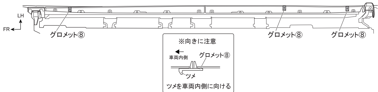
図3 下面視 ※LH図示 左右共通作業
