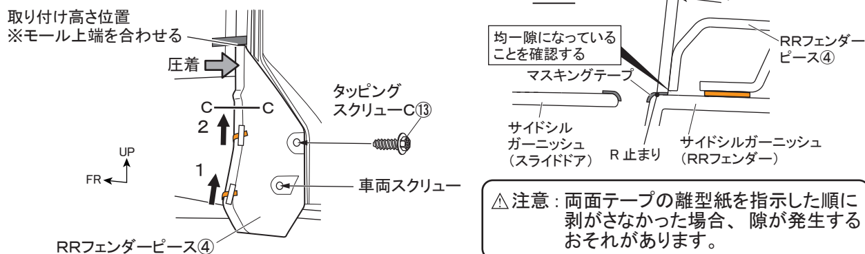
図 29 ※LH図示 左右共通作業
