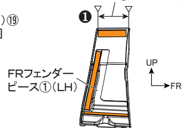
モール（イ型）⑩貼り付け範囲
