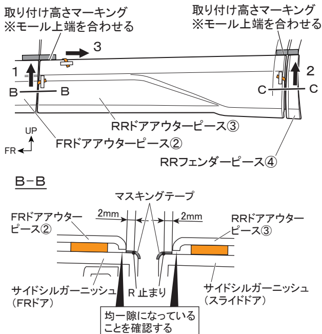
図 32 ※LH図示 左右共通作業
