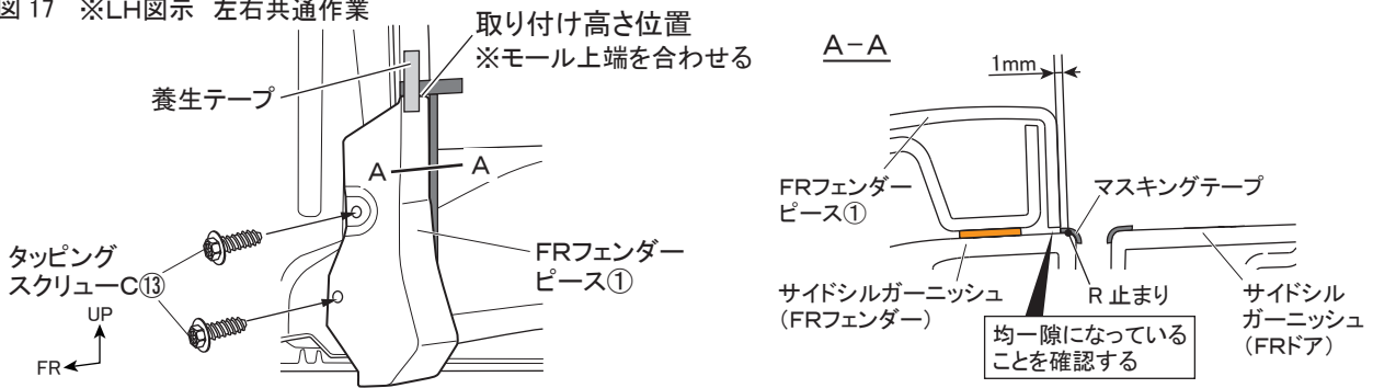
図 17 ※LH図示 左右共通作業
