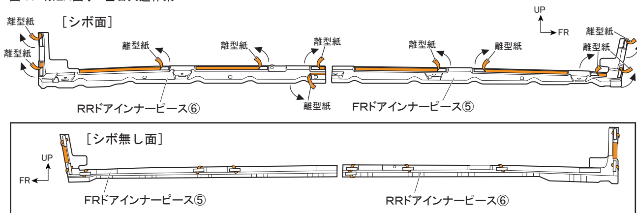
図11 ※LH図示 左右共通作業
