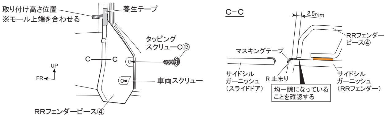
図 18 ※LH図示 左右共通作業
