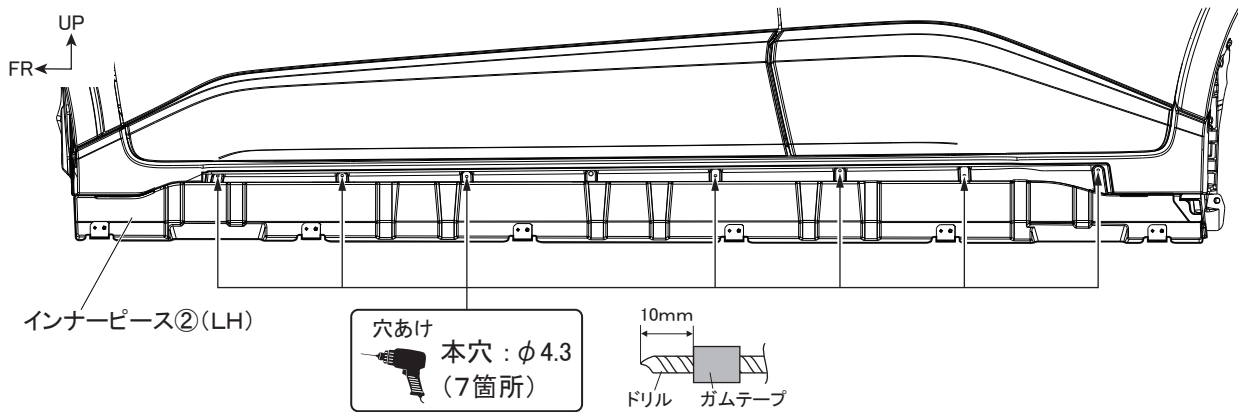
図 15 ※LH図示 左右共通作業
