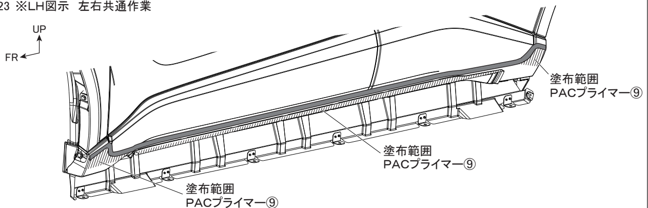
図 23 ※LH図示 左右共通作業
