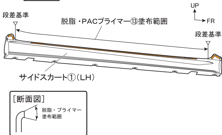
図3 裏面視 ※LH図示 左右共通作業
