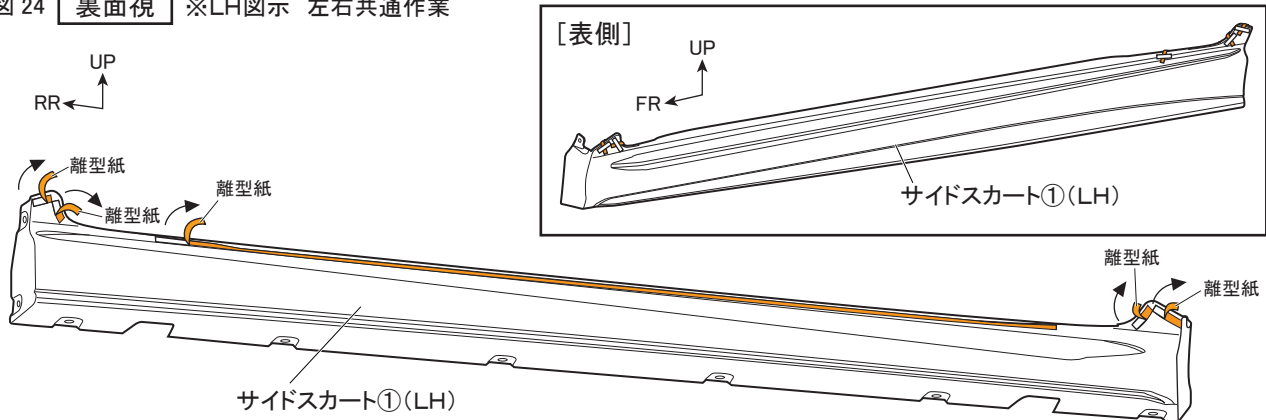
図 24 裏面視 ※LH図示 左右共通作業
