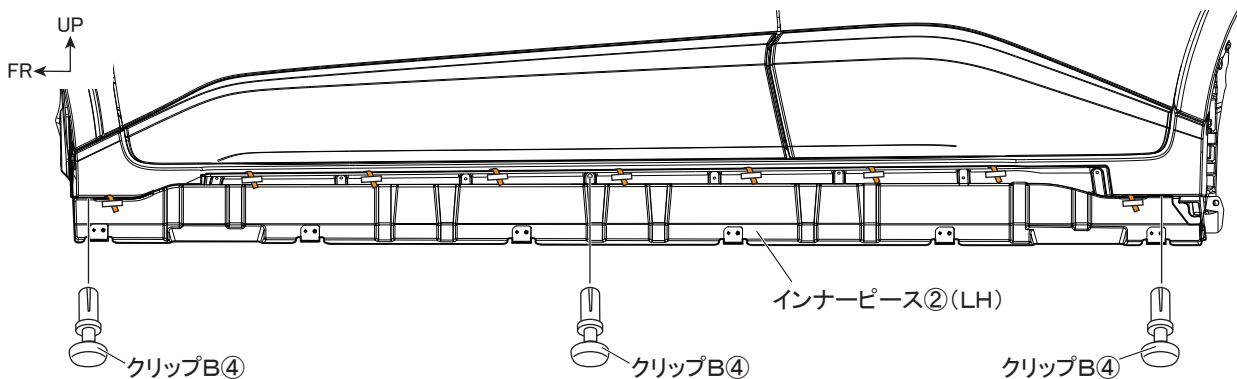
図 13 ※LH図示 左右共通作業
