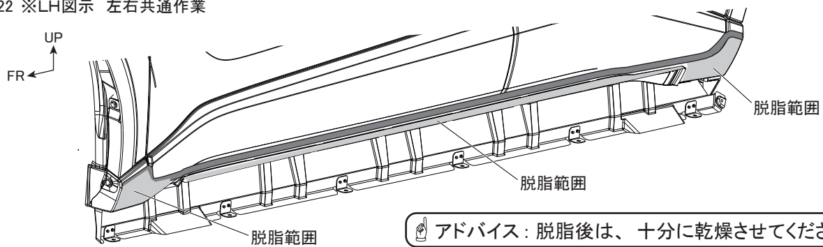
図 22 ※LH図示 左右共通作業
