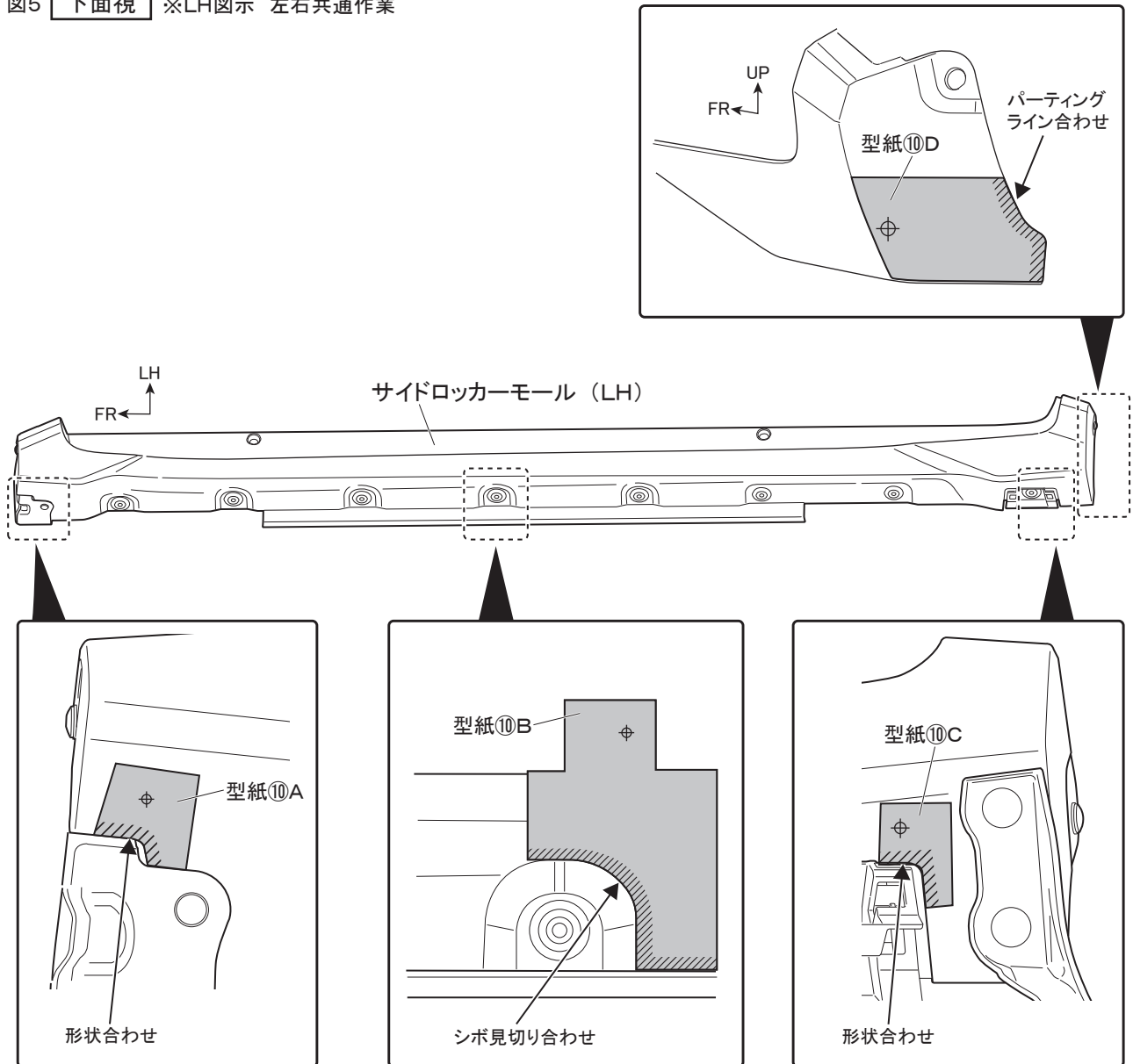
図5 下面視 ※LH図示 左右共通作業
