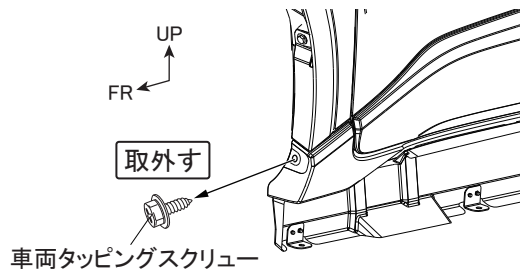
図 17 ※LH図示 左右共通作業
