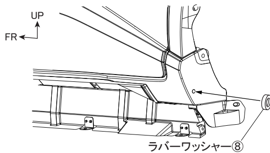
図 19 ※LH図示 左右共通作業
