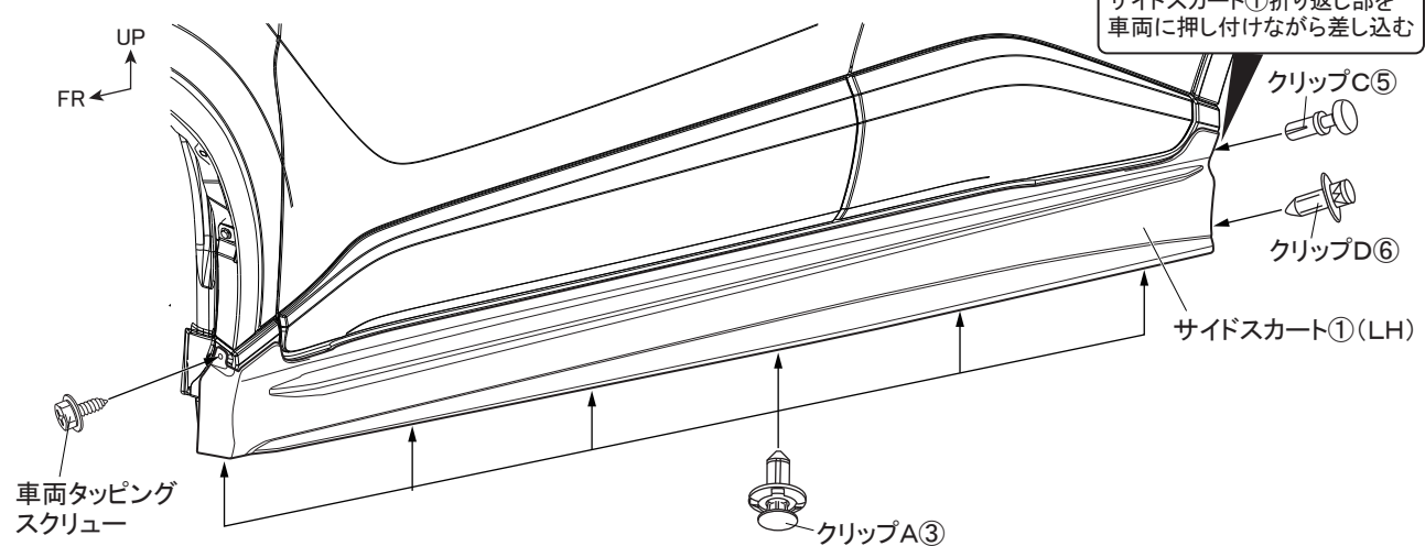
図 20 ※LH図示 左右共通作業
