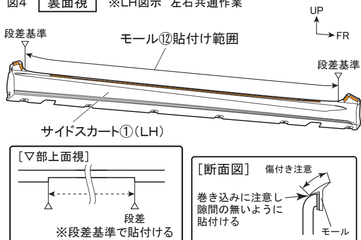
図4 裏面視 ※LH図示 左右共通作業
