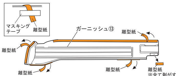
図 14 ※LH図示 左右共通作業
