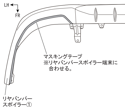
下面視
