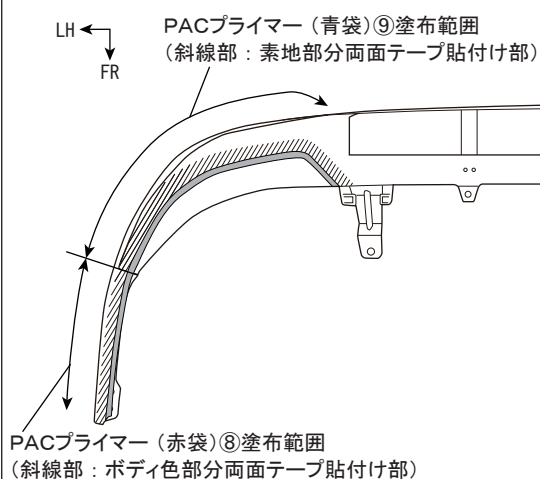
下面視
