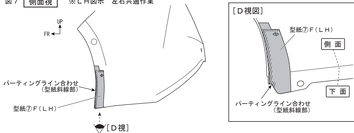
図 7 側面視 ※ L H 図示 左右共通作業
