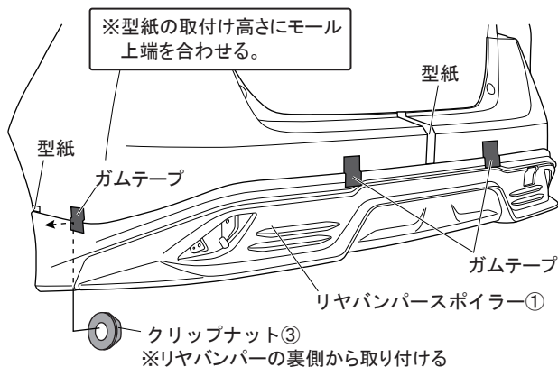
図 16 ※LH図示 左右共通作業
