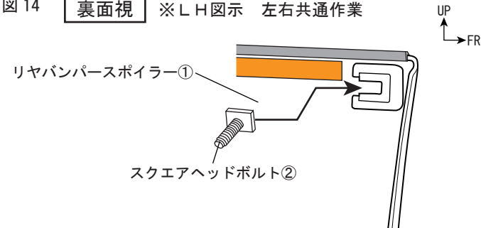
図 14 裏面視 ※LH図示 左右共通作業
