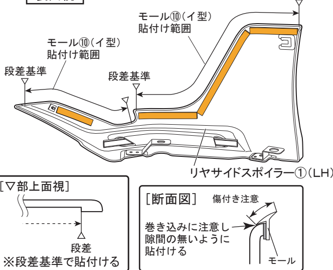
図4 裏面視 ※LH図示 左右共通作業
