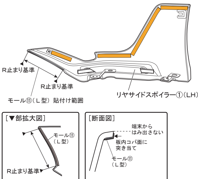
図5 裏面視 ※LH図示 左右共通作業
