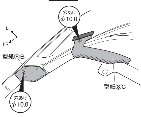
<B視拡大図> 下面視
