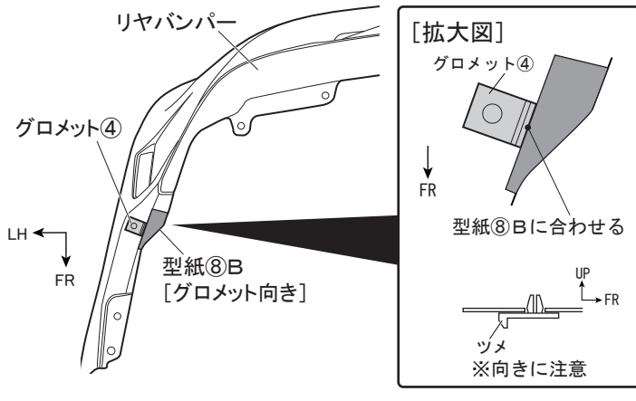
図 18 裏面視 ※LH図示 左右共通作業
