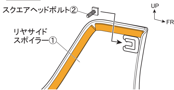
図 18 裏面視 ※LH図示 左右共通作業
