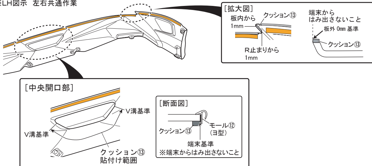
図5 ※LH図示 左右共通作業
