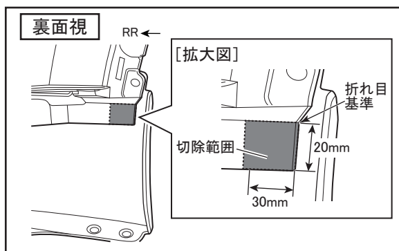
図 14 ※LH図示 左右共通作業
