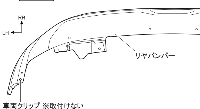
図 15 下面視 ※LH図示 左右共通作業
