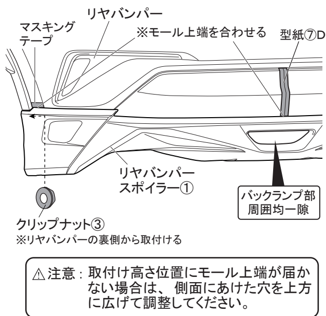
図 17 ※LH図示 左右共通作業
