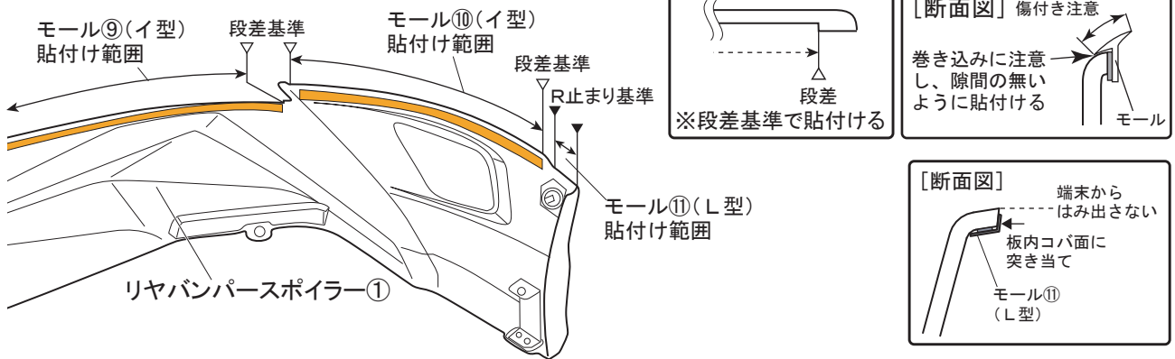
図3 裏面視 ※LH図示 左右共通作業
