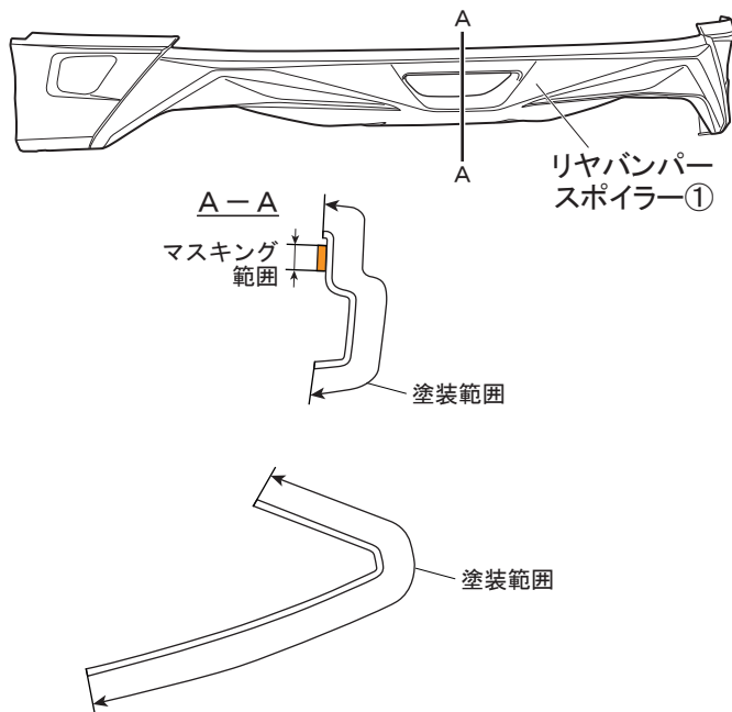
図1 ※LH図示 左右共通作業
