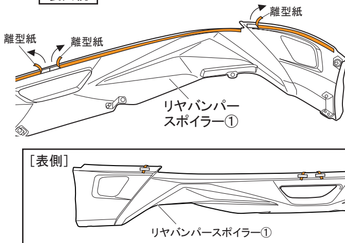
図 21 裏面視 ※LH図示 左右共通作業
