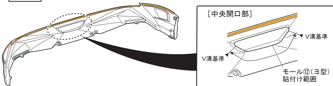
図4 裏面視 ※LH図示 左右共通作業
