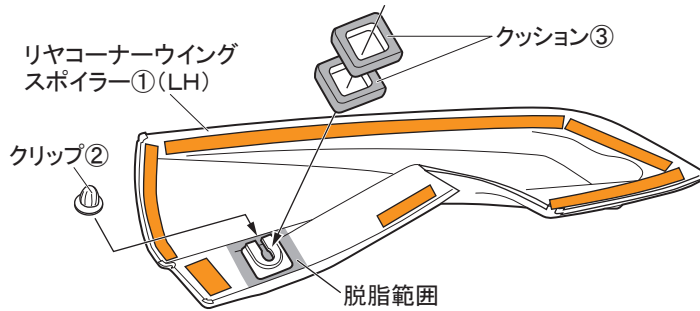
図6 裏面視 ※LH図示 左右共通作業
