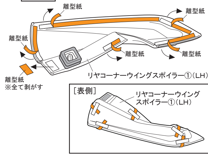
図 10 裏面視 ※LH図示 左右共通作業
