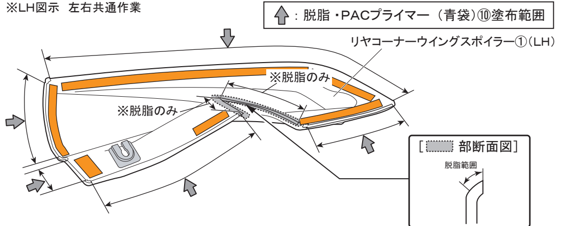
図2 裏面視 ※LH図示 左右共通作業
