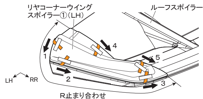
図 11 ※LH図示 左右共通作業
