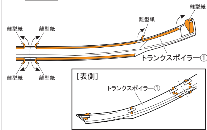
図7 裏面視 ※LH図示 左右共通作業
