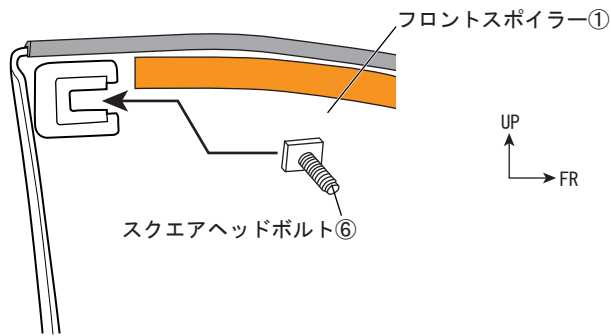
図 13 裏面視 ※LH図示 左右共通作業
