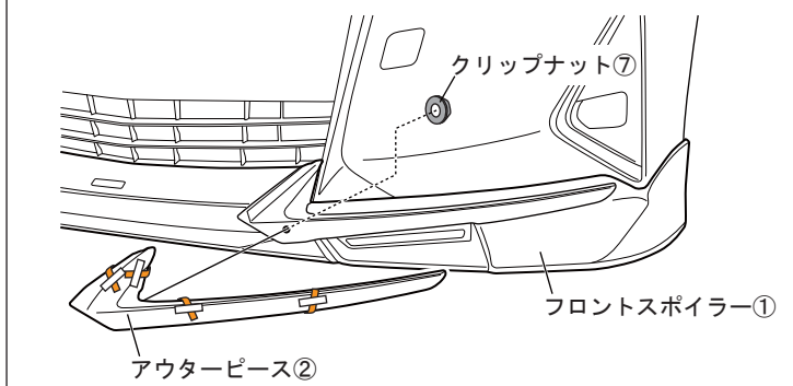
図 20 ※LH図示 左右共通作業
