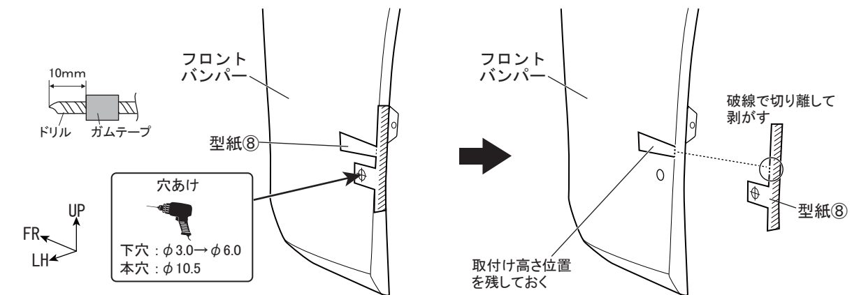
図7 ※LH図示 左右共通作業
