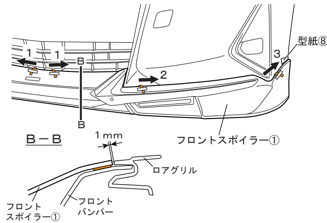
図 16 ※LH図示 左右共通作業
