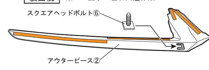
図 18 裏面視 ※LH図示 左右共通作業
