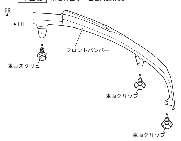
図8 下面視 ※LH図示 左右共通作業
