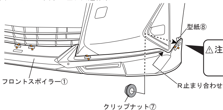
図 15 ※LH図示 左右共通作業
