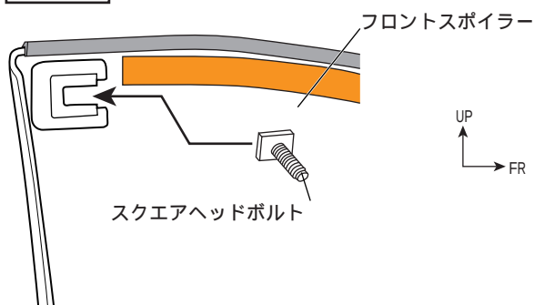
図 13 裏面視 L H図示 左右共通作業
