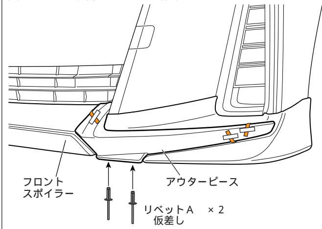
図 19 L H 図示 左右共通作業
