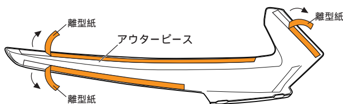
図 18 裏面視 L H 図示 左右共通作業
