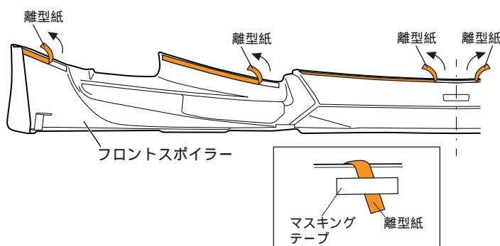
図 14 裏面視 L H図示 左右共通作業
