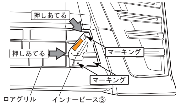
図 12 ※LH図示 左右共通作業
