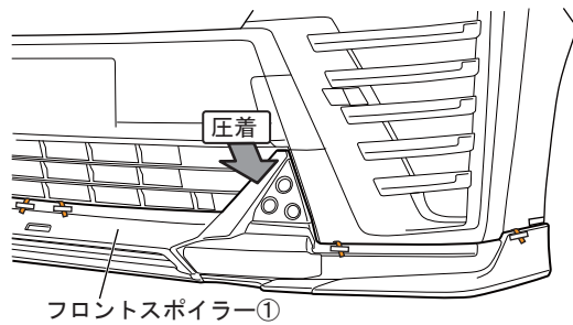
図 23 ※L H図示 左右共通作業
