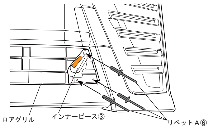
図 14 ※LH図示 左右共通作業
