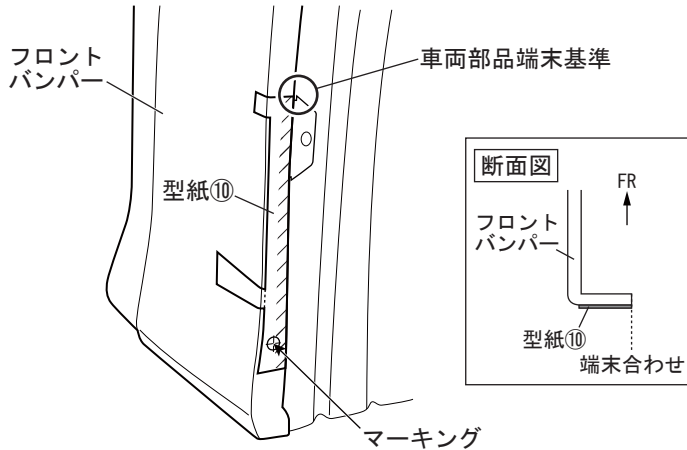
図 9 ※LH図示 左右共通作業
