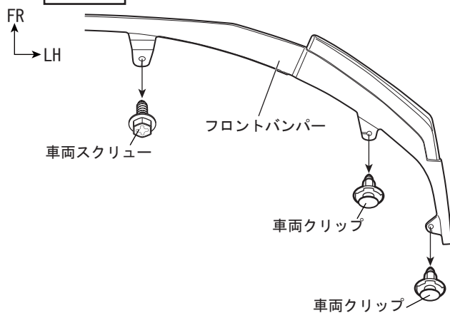
図 15 下面視 ※LH図示 左右共通作業
