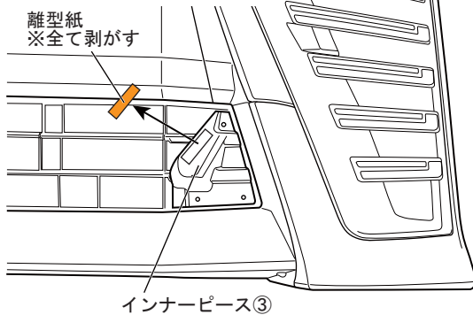
図 20 ※ L H 図示 左右共通作業
