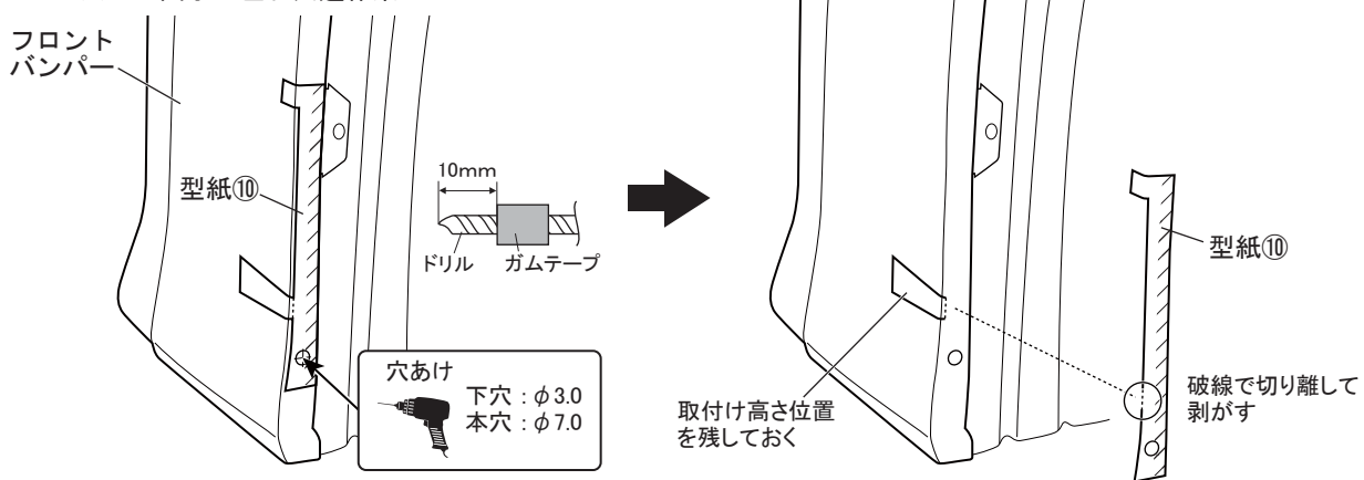
図 10 ※LH図示 左右共通作業
