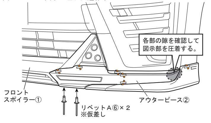
図 26 ※L H図示 左右共通作業
