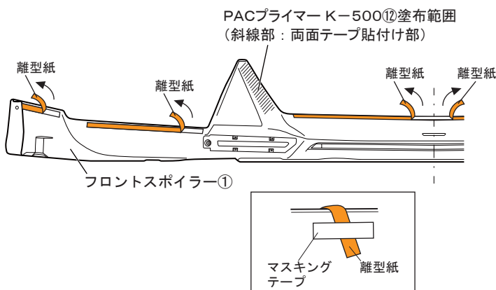
図 21 裏面視 ※ L H 図示 左右共通作業
