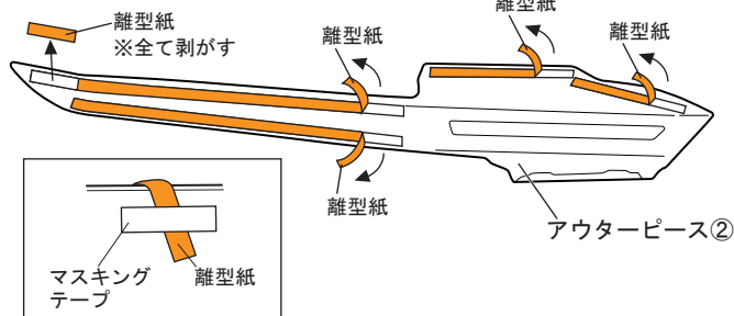
図 25 ※L H図示 左右共通作業
