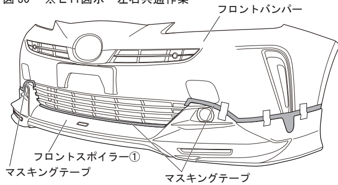
図 30 ※LH図示 左右共通作業
