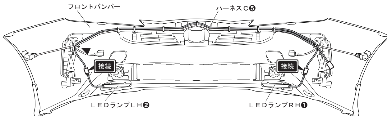
図 35 裏面視 ※図は I C S 装着車です。非装着車も同様に作業してください。
