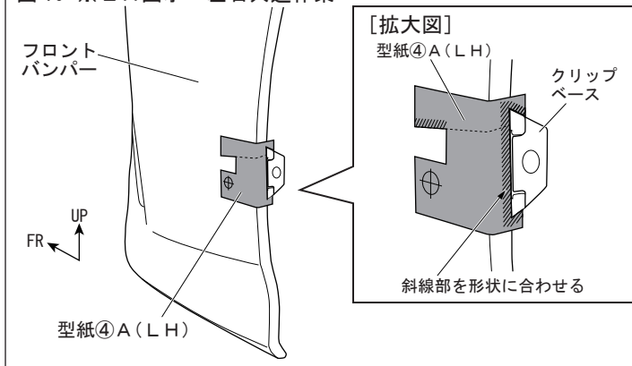
図 10 ※LH図示 左右共通作業
