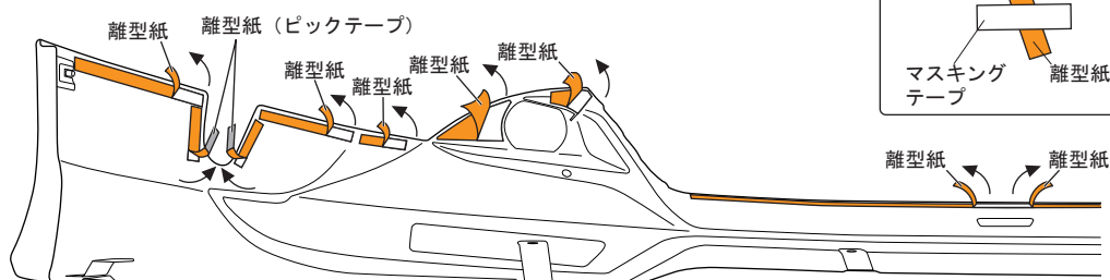
図 33 ※LH図示 左右共通作業
