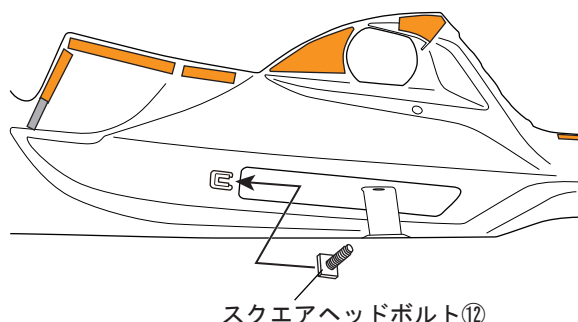
図8 ※LH図示 左右共通作業
