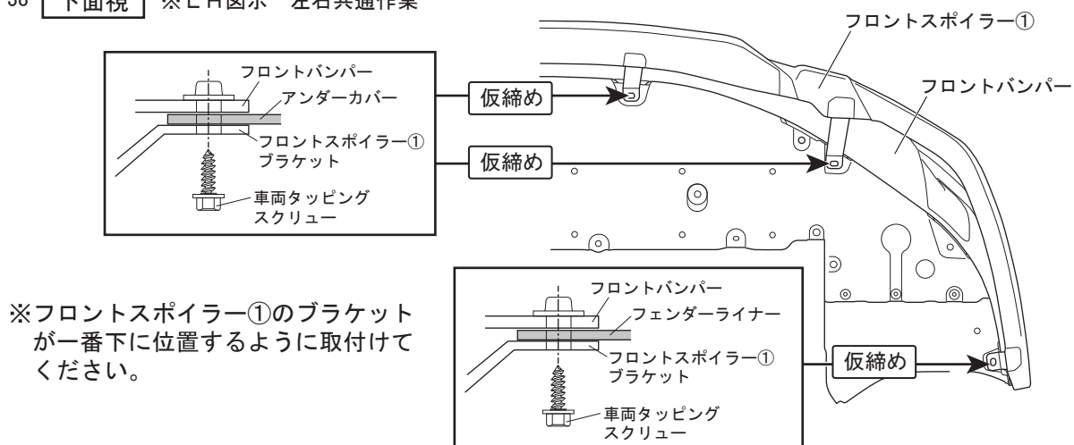
図 38 下面視 ※LH図示 左右共通作業
