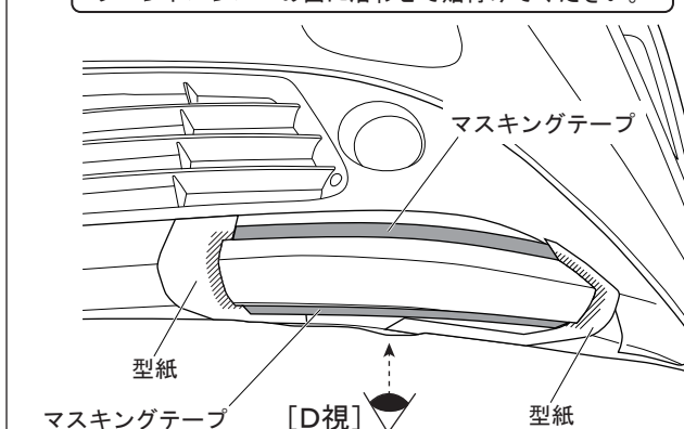
図 12 ※LH図示 左右共通作業
