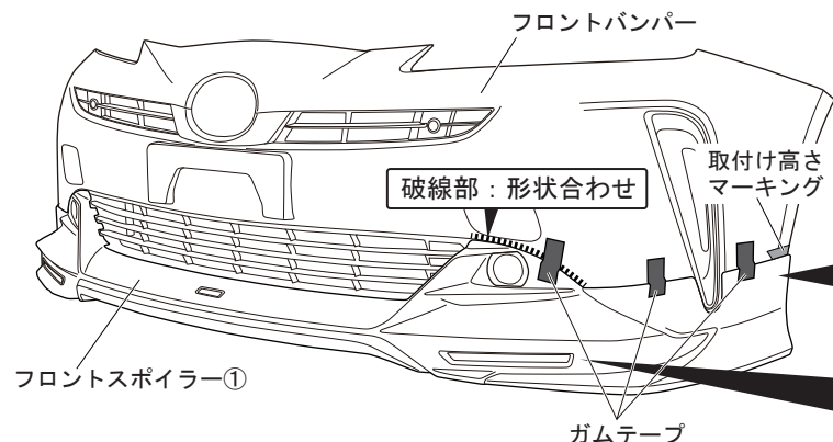
図 29 ※LH図示 左右共通作業
