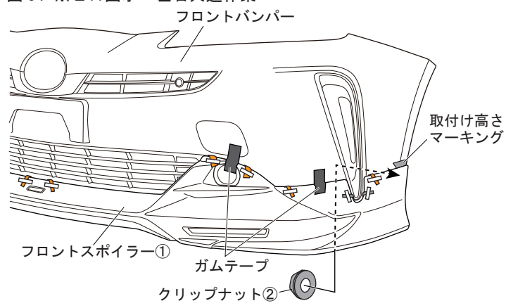
図 34 ※LH図示 左右共通作業
