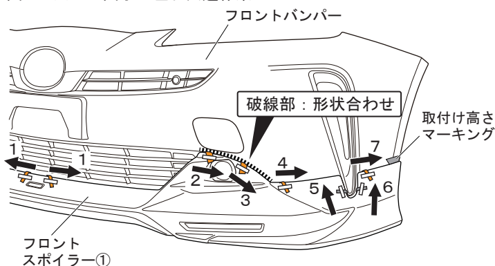
図 39 ※LH図示 左右共通作業
