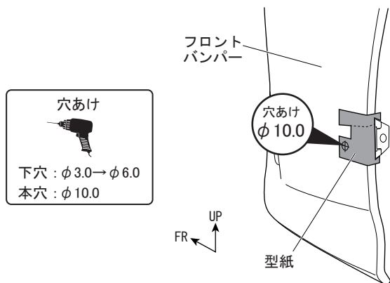
図 14 ※LH図示 左右共通作業
