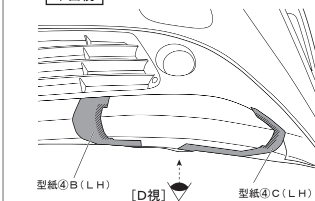
図 11 下面視 ※LH図示 左右共通作業
