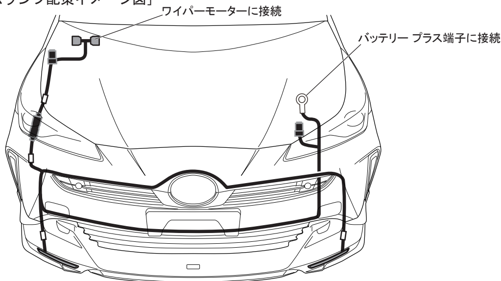
[LEDデイトタイムランプ配線イメージ図]
