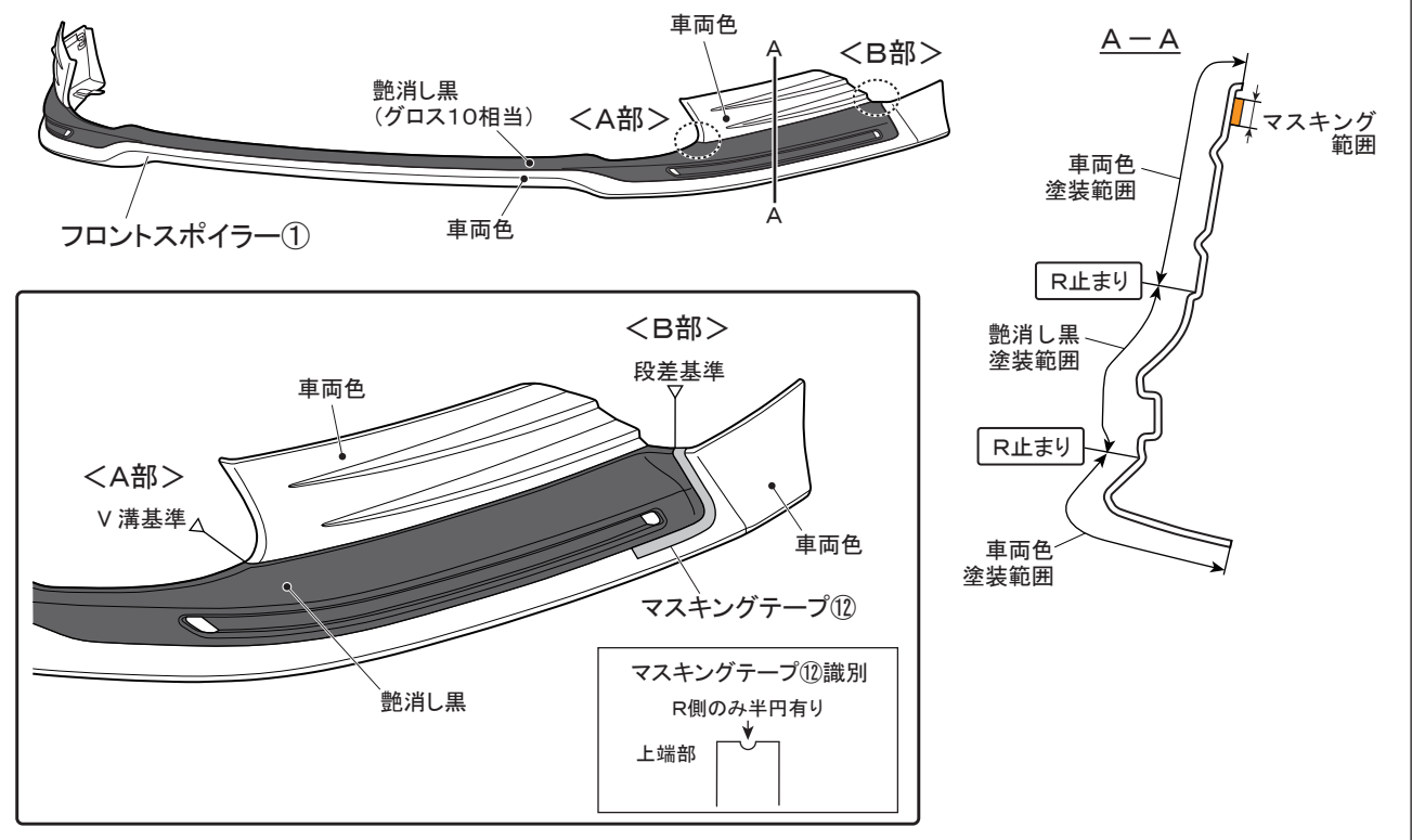
図2 ※LH図示 左右共通作業
