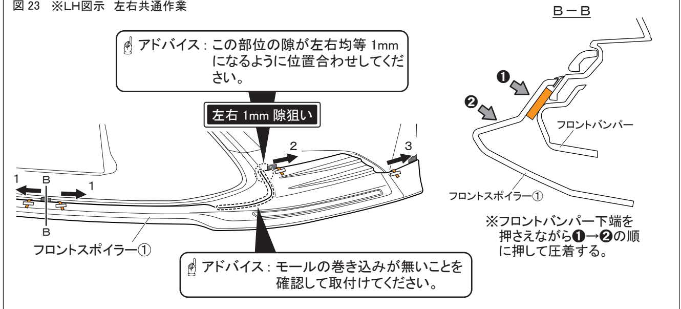
図 23 ※LH図示 左右共通作業
