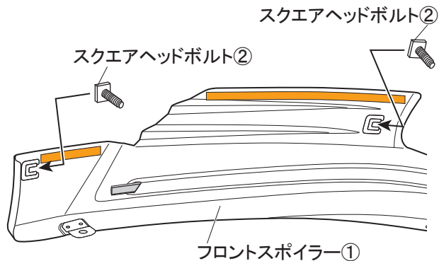
図 15 裏面視 ※LH図示 左右共通作業
