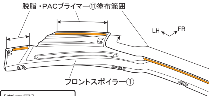
図3 裏面視 ※LH図示 左右共通作業
