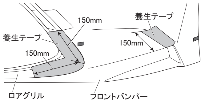
図 16 ※LH図示 左右共通作業
