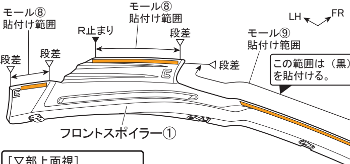
図4 裏面視 ※LH図示 左右共通作業
