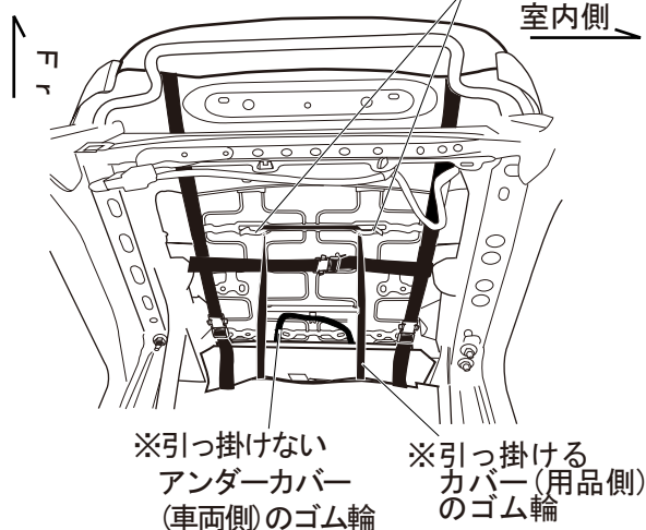
〈シートクッション裏側図〉
