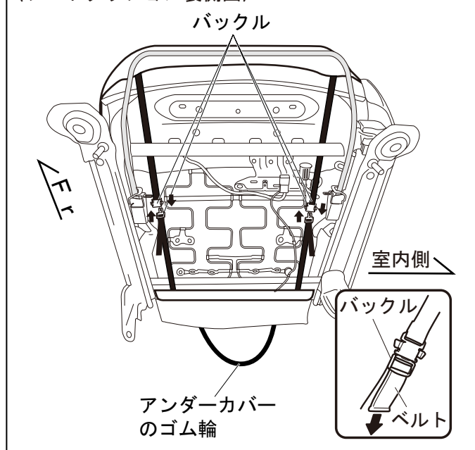
〈シートクッション裏側図〉
