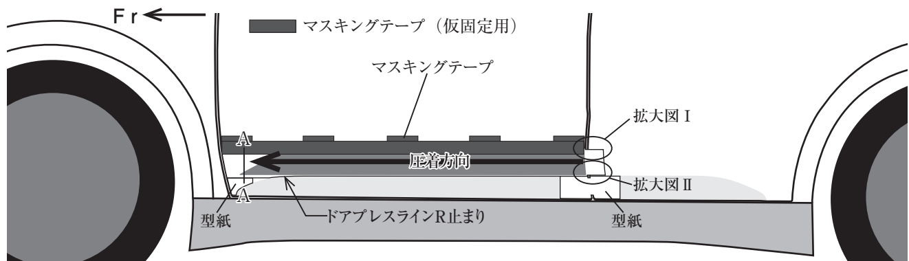
図1 LHFr ドア図
