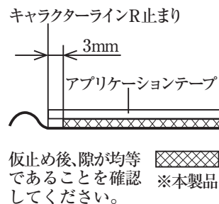
B-B 断面図
