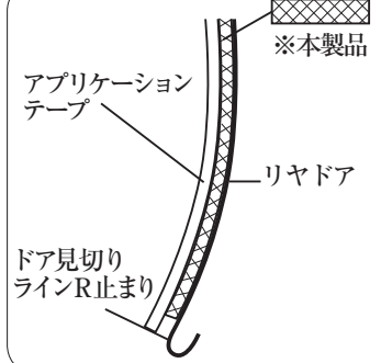
B-B断面図
