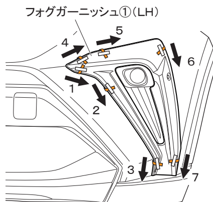
図9 ※LH図示 左右共通作業
