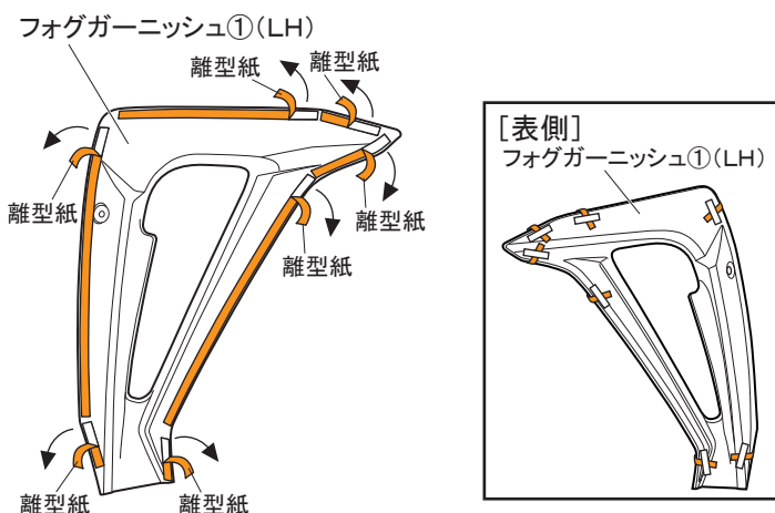
図7 裏面視 ※LH図示 左右共通作業
