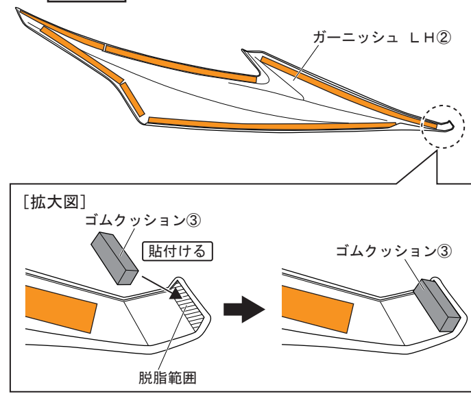
図1 裏面視 ※LH図示 左右共通作業
