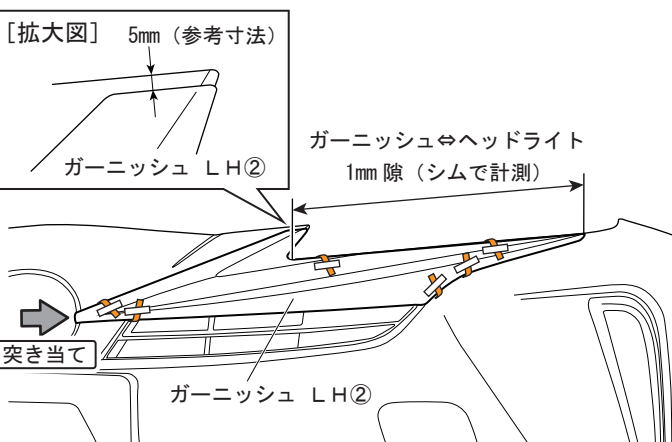
図7 ※LH図示 左右共通作業
