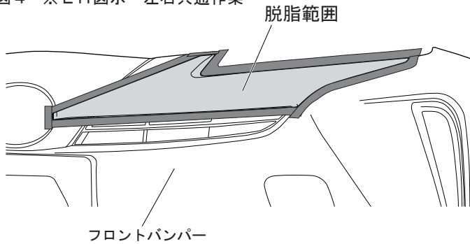
図4 ※LH図示 左右共通作業
