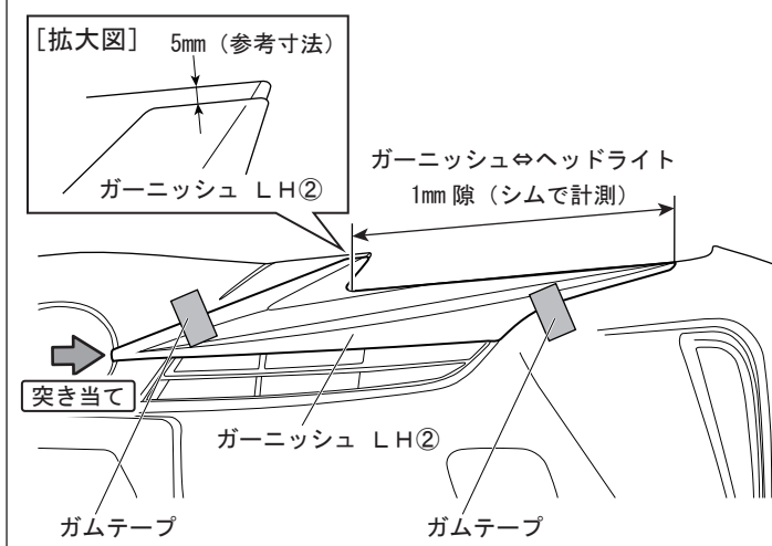
図2 ※LH図示 左右共通作業
