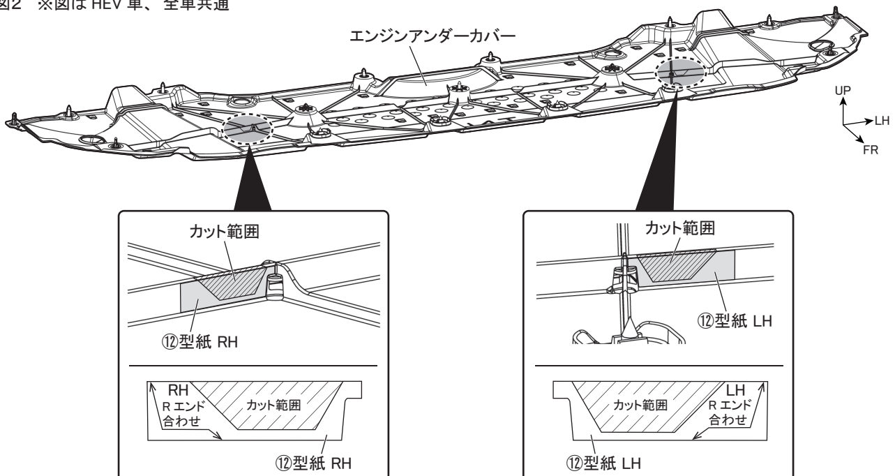
図2 ※図は HEV 車、全車共通
