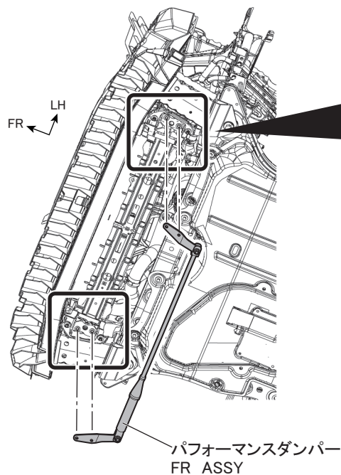
図5 下面視 ※図は HEV 車、全車共通
