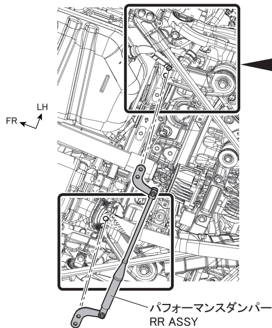
図 13 下面視 ※図は 4WD 車、2WD 車も共通
