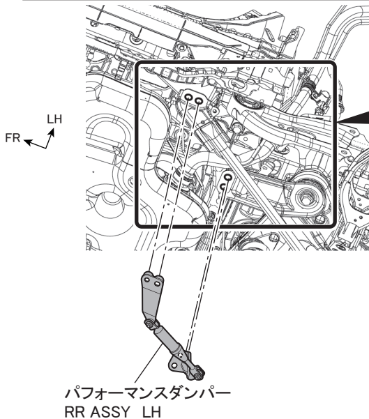
図9 下面視 ※LH図示 左右共通作業
