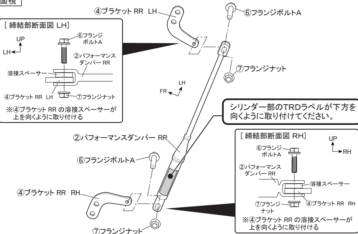
図 12 下面視
