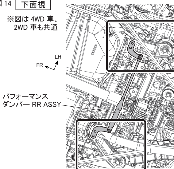
図 14 下面視
