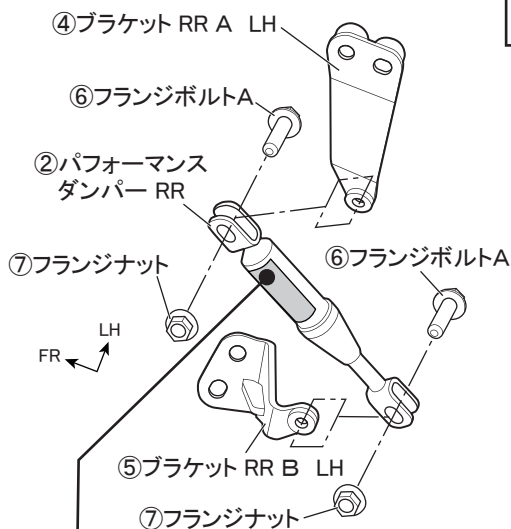
図8 下面視 ※LH図示 左右共通作業
