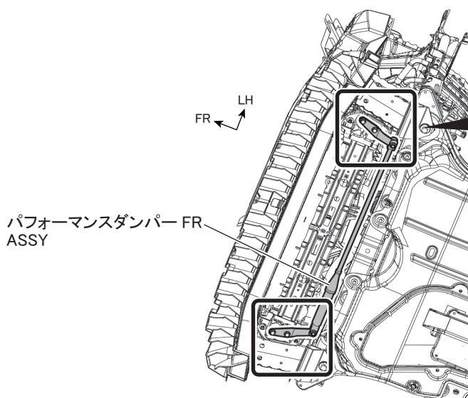
図6 下面視 ※図は HEV 車、全車共通
