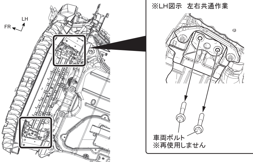
図3 下面視 ※図は HEV 車、全車共通
