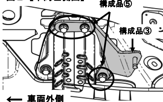
図2 【車両左側図】
