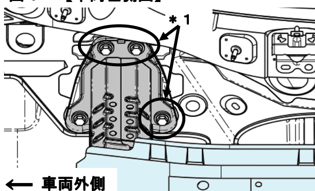
図1 【車両左側図】
