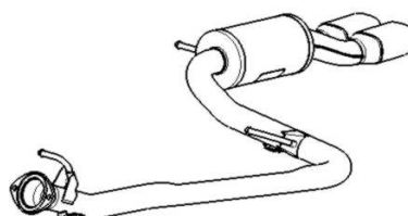
①GRドレスアップマフラー (MS153-58014)
