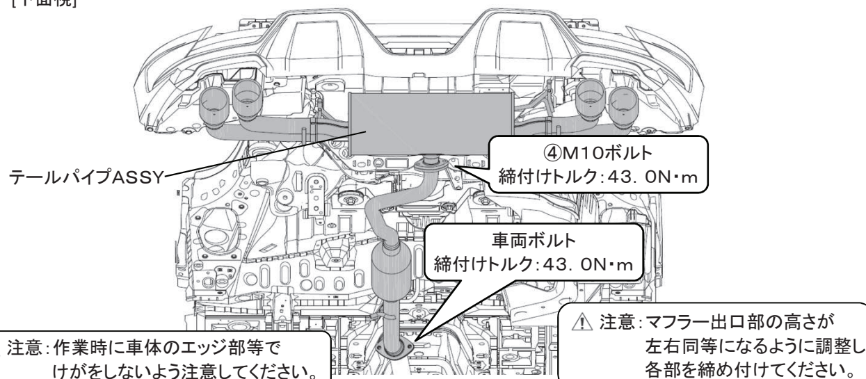
図3 [下面視]
