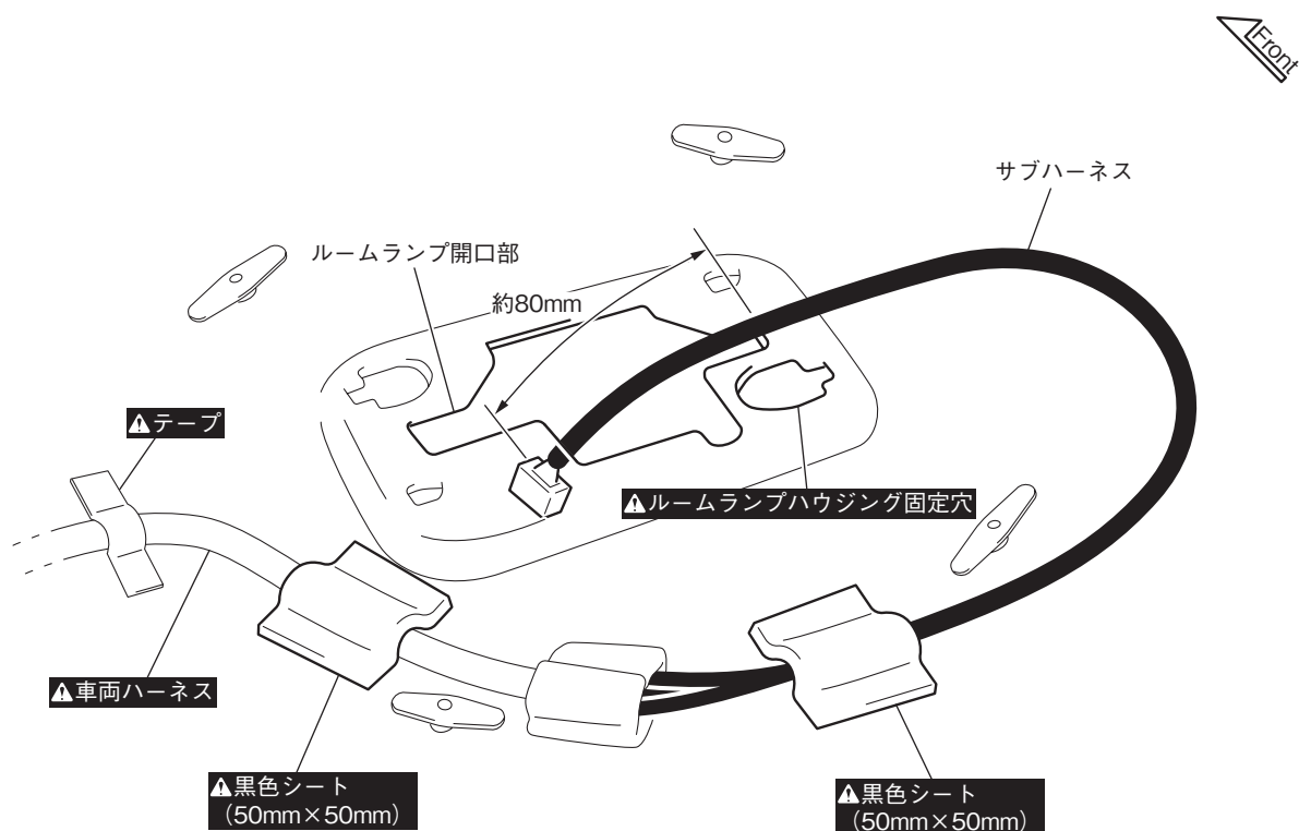
ルーフヘッドライニング裏側の詳細図
