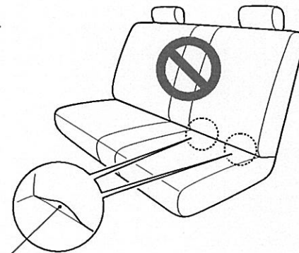
ISOFIX対応チャイルドシート固定専用バーがない
